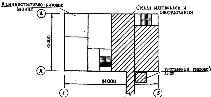
Схема привязки объекта ГО
