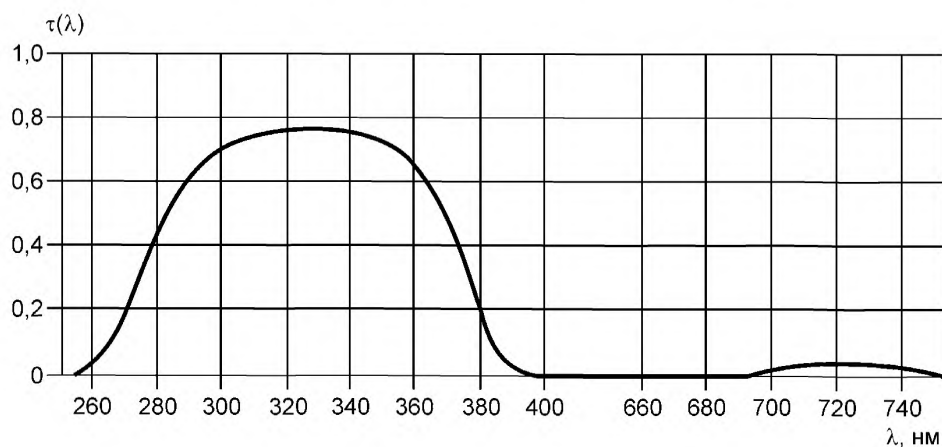
Рисунок 3 — Спектральный коэффициент пропускания \tau(\lambda) корректирующего УФ-фильтра
