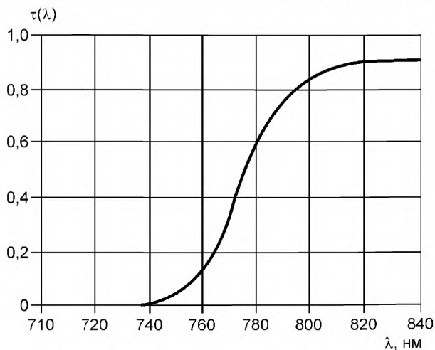
Рисунок 4 — Спектральный коэффициент пропускания \tau(\lambda) корректирующего ИК-фильтра
