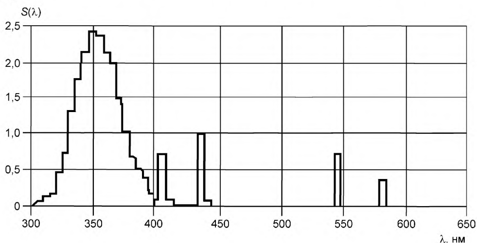
Рисунок 2 — Спектральное распределение излучения лампы
