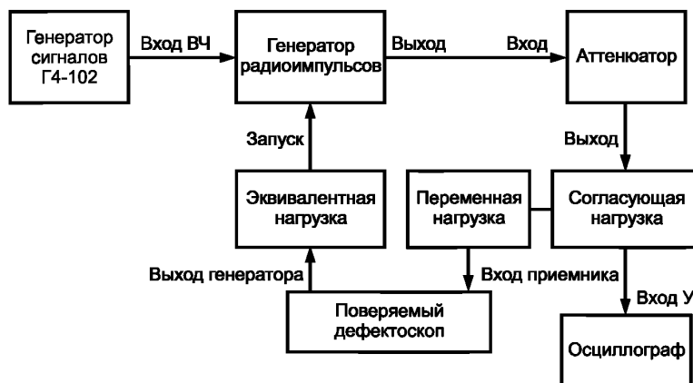
Рисунок 1 — Схема установки для проверки дефектоскопов
