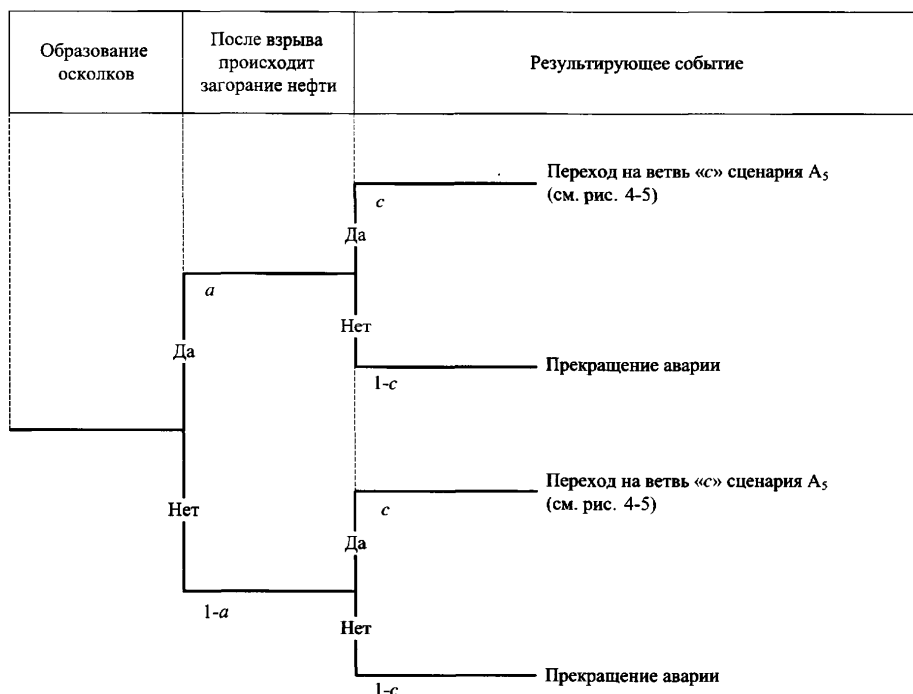
Рис. 4-6. Дерево событий при взрыве внутри подземного резервуара (типа ЖБР) (сценарий A_6 )
