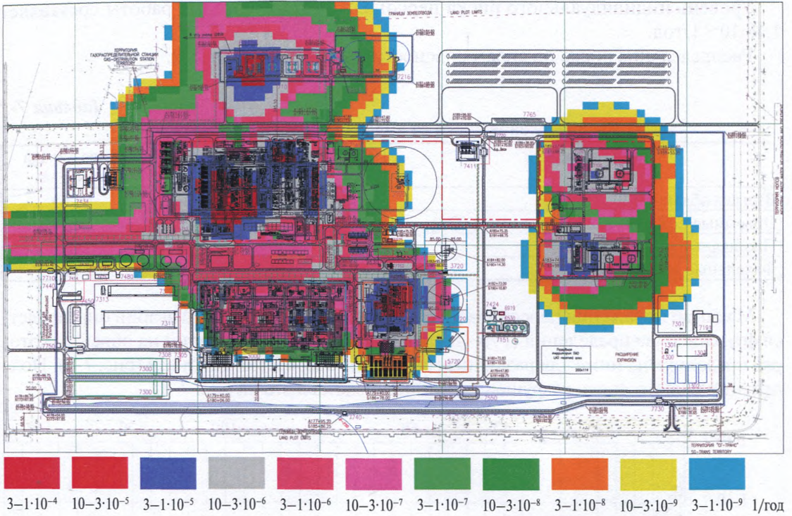
Рис. 7-2. Территориальное распределение превышения избыточного давления во фронте УВ (120 кПа) для сценариев Впю на объекте
