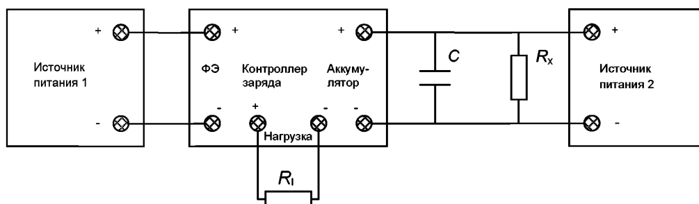
Рисунок 3 — Схема проверки без подключения измерительных приборов
