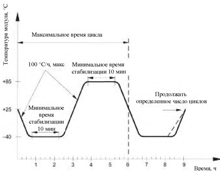
Рисунок 4 — Термоциклирование
