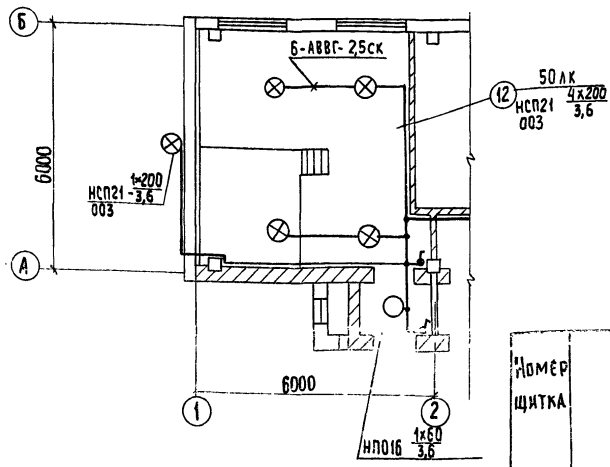
ВАРИАНТ С ХЛОРОДОЗАТОРНОЙ
