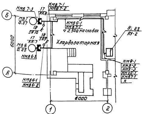
Элемент плана на отм. 0.000.
