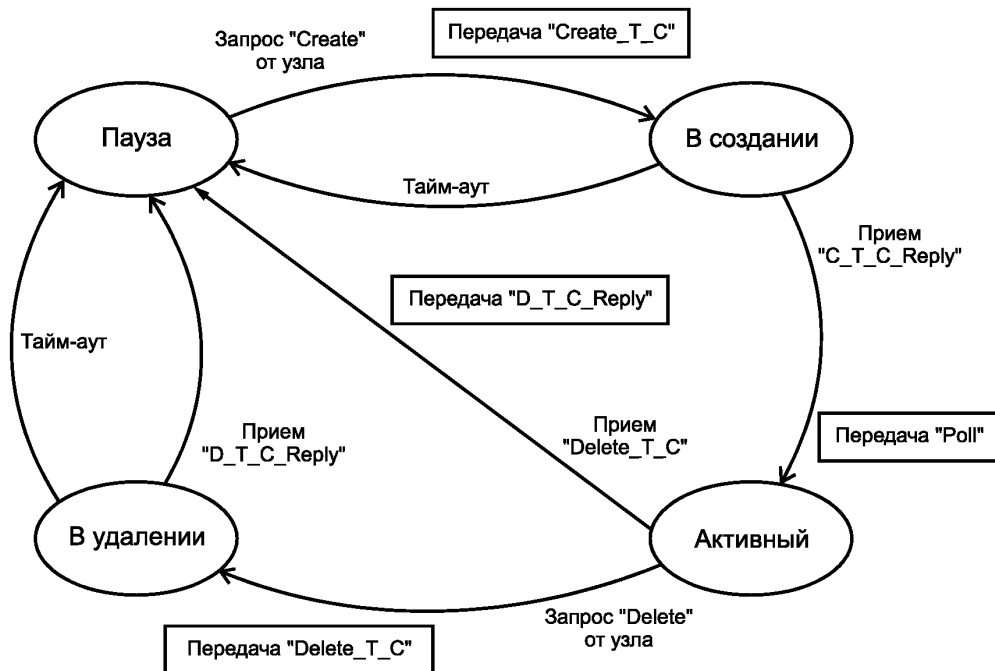
Рисунок 5 — Диаграмма состояний транспортного протокола на узле
