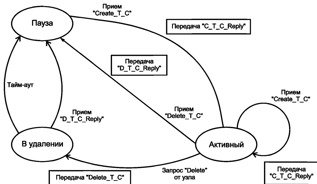
Рисунок 6 — Диаграмма состояний транспортного протокола на модуле
