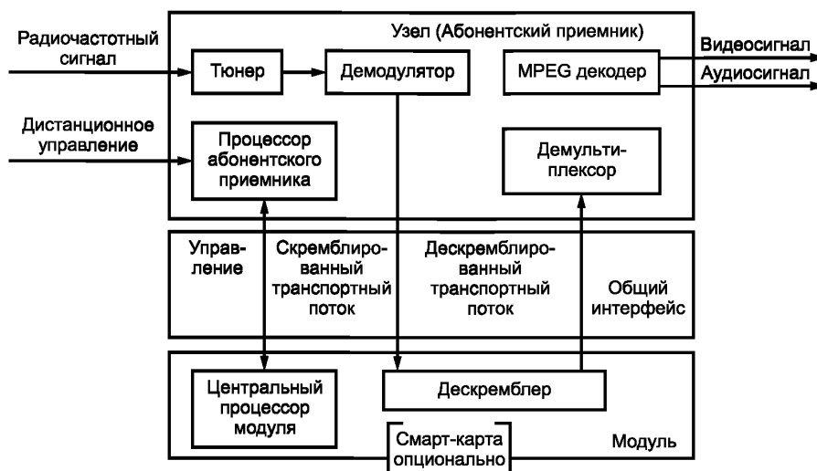
Рисунок 1 — Структурная схема приемного оборудования СОД
