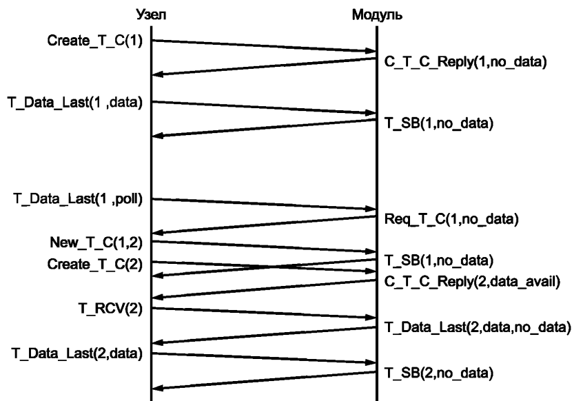
Рисунок 7 — Пример передачи объектов транспортного протокола
