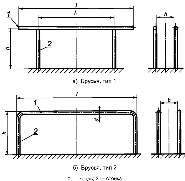
Рисунок 3 — Параллельные брусья
