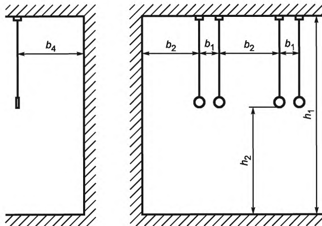
Рисунок 6 — Установочные размеры для колец
