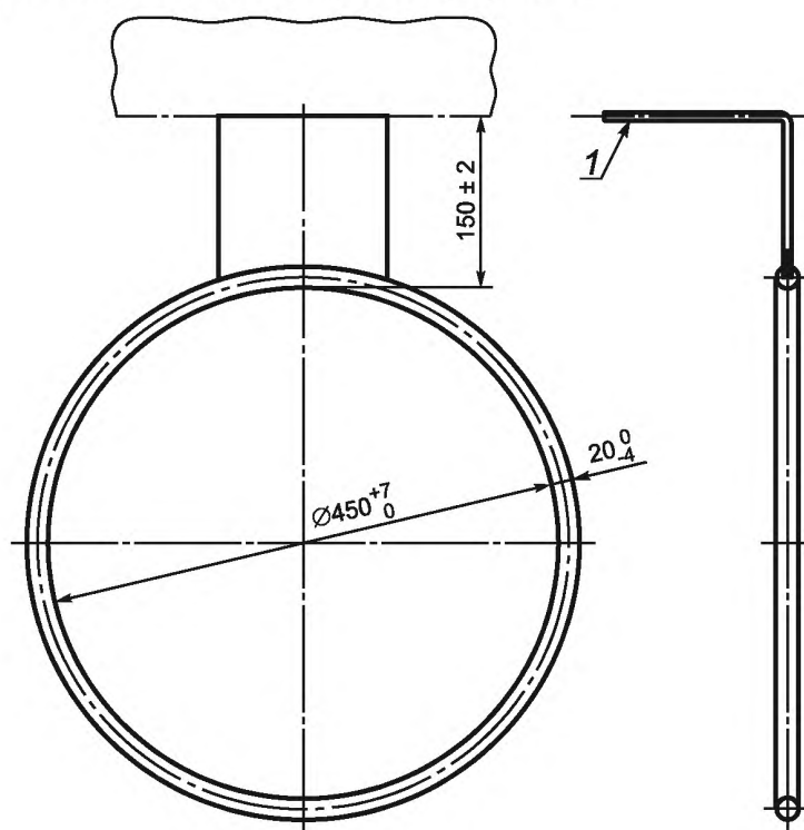
Рисунок 11 — Размеры баскетбольного кольца
