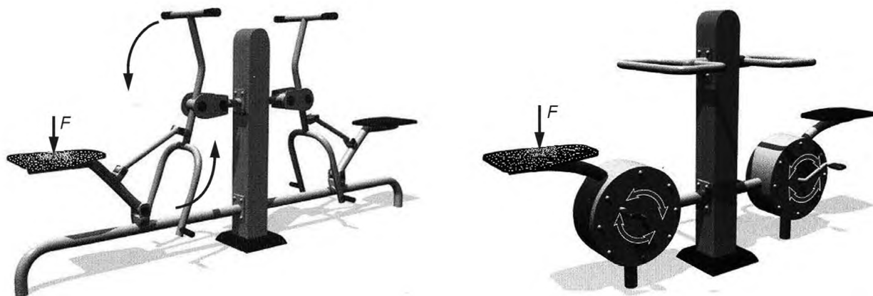
Рисунок Е.3 — Примеры приложения нагрузки
