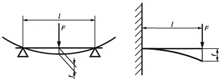
Рисунок 9 — Пример нагружения элементов тренажера
