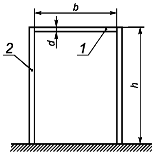
Рисунок 2 — Перекладина
