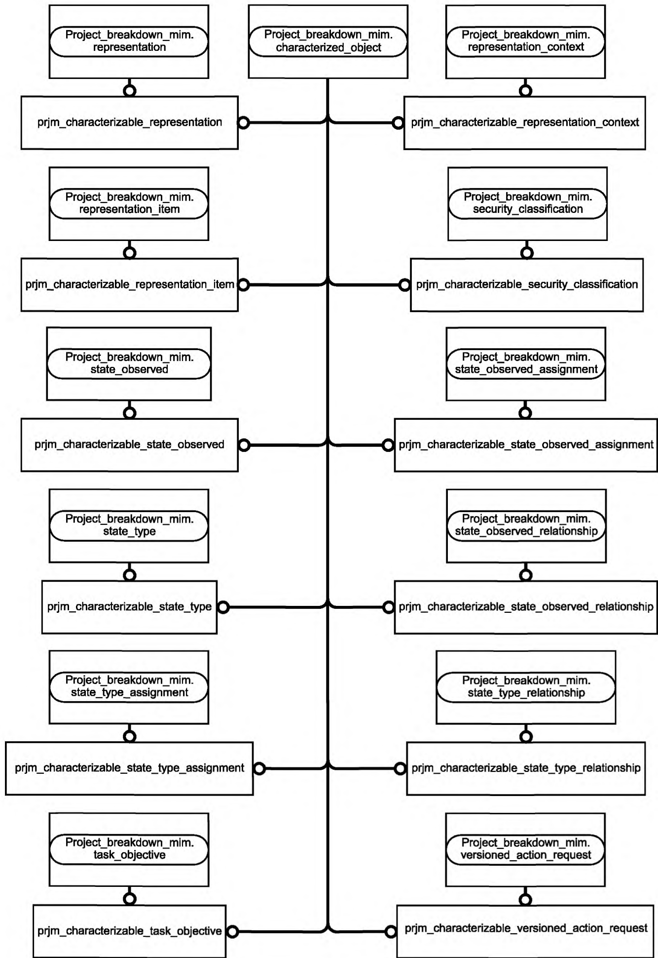
Рисунок D.3 — Представление IMM на уровне объектов в формате EXPRESS-G (диаграмма 2 из 2)
