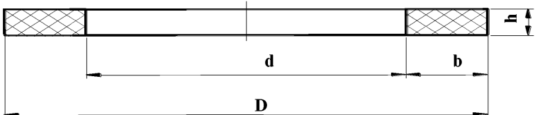
Рисунок В.4 – Конструкция колец графитовых уплотнительных КГУ по ТУ 38.314-25-3-91
