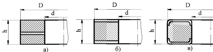
Рисунок В.7 – Конструкции колец армированных графитовых уплотнительных КАГУ: а) тип 1; б) тип 2; в) тип 3.
