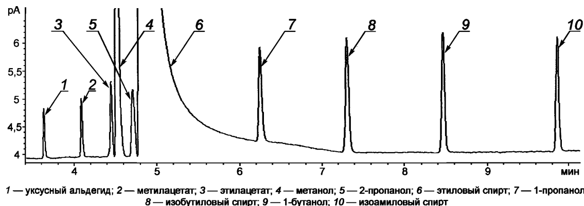
Рисунок 1 — Хроматограмма анализа градуировочной смеси, полученная на хроматографе, оснащённом капиллярной колонкой
