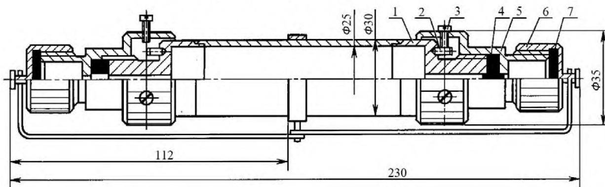
Рисунок 8 — Пробоотборник ПУ-400
