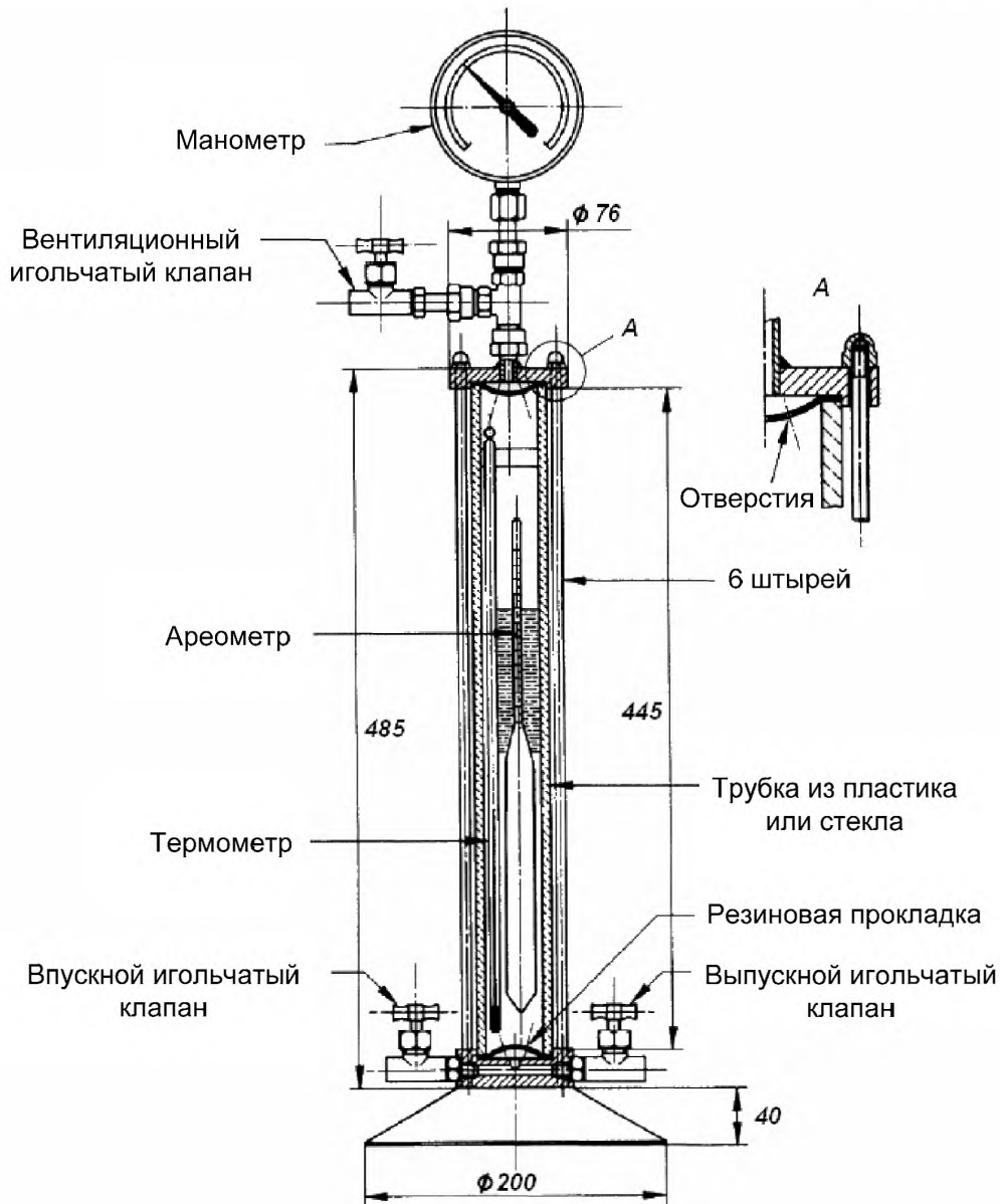
Рисунок 13 — Ареометр давления
