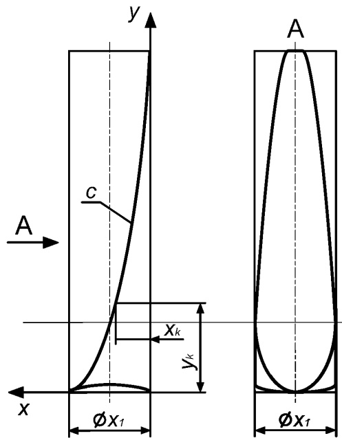
Рисунок 5— Стабилизатор
