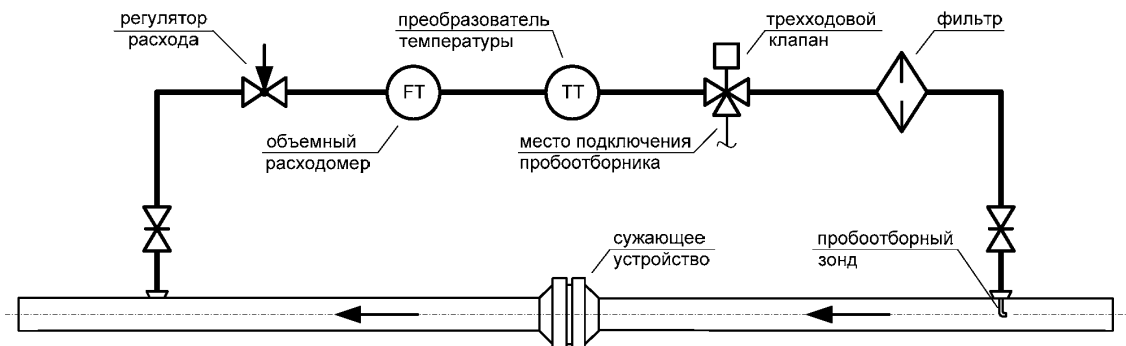
Рисунок 6 — Схема отбора проб с помощью сужающего устройства
