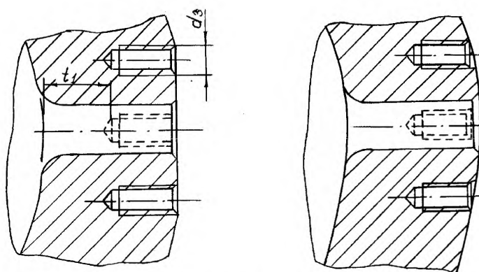
Рисунок 4.4 – Размещение резьбовых гнезд для крепежных элементов
