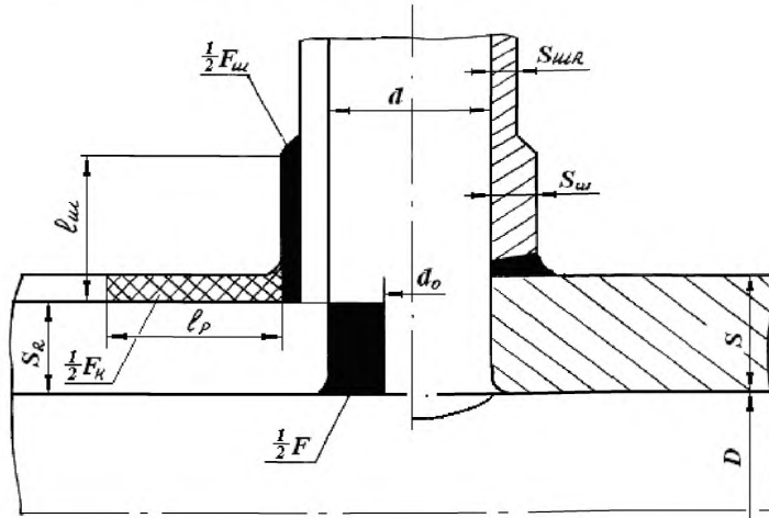
Рисунок 5.1 – Схема компенсации площадей при укреплении отверстия
