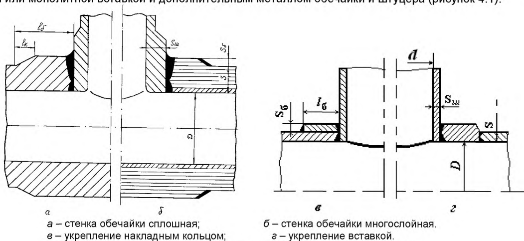
Рисунок 4.1 – Способы укрепления отверстий в обечайке (днище)
