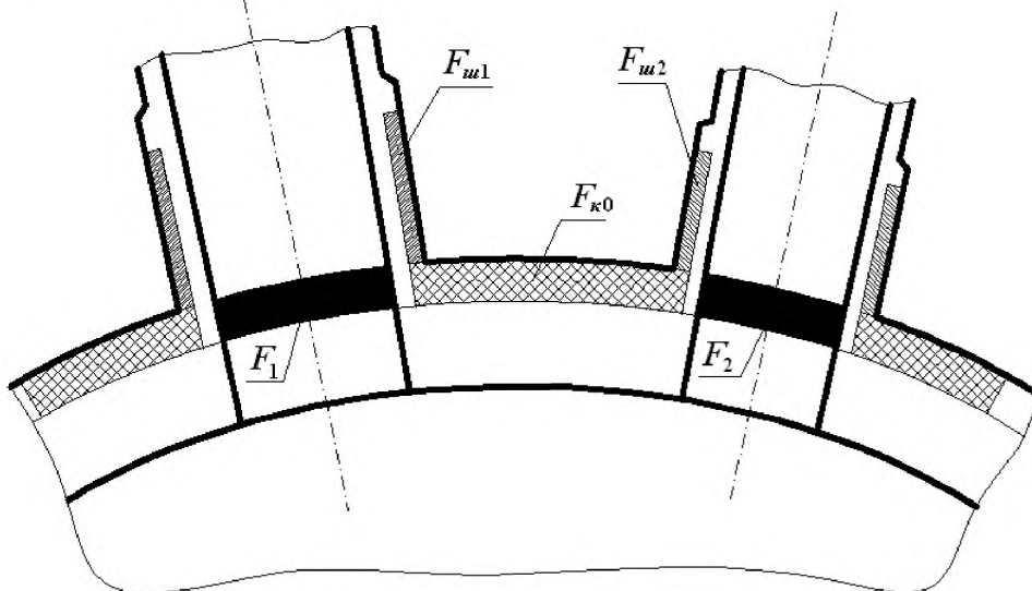
Рисунок 5.2 – Схема укрепления взаимовлияющих отверстий
