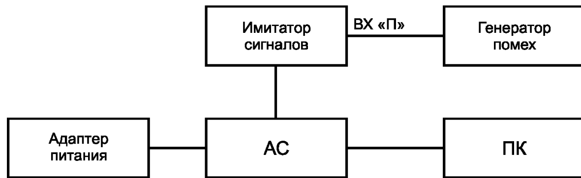
Рисунок Д.5 — Схема испытательного стенда
