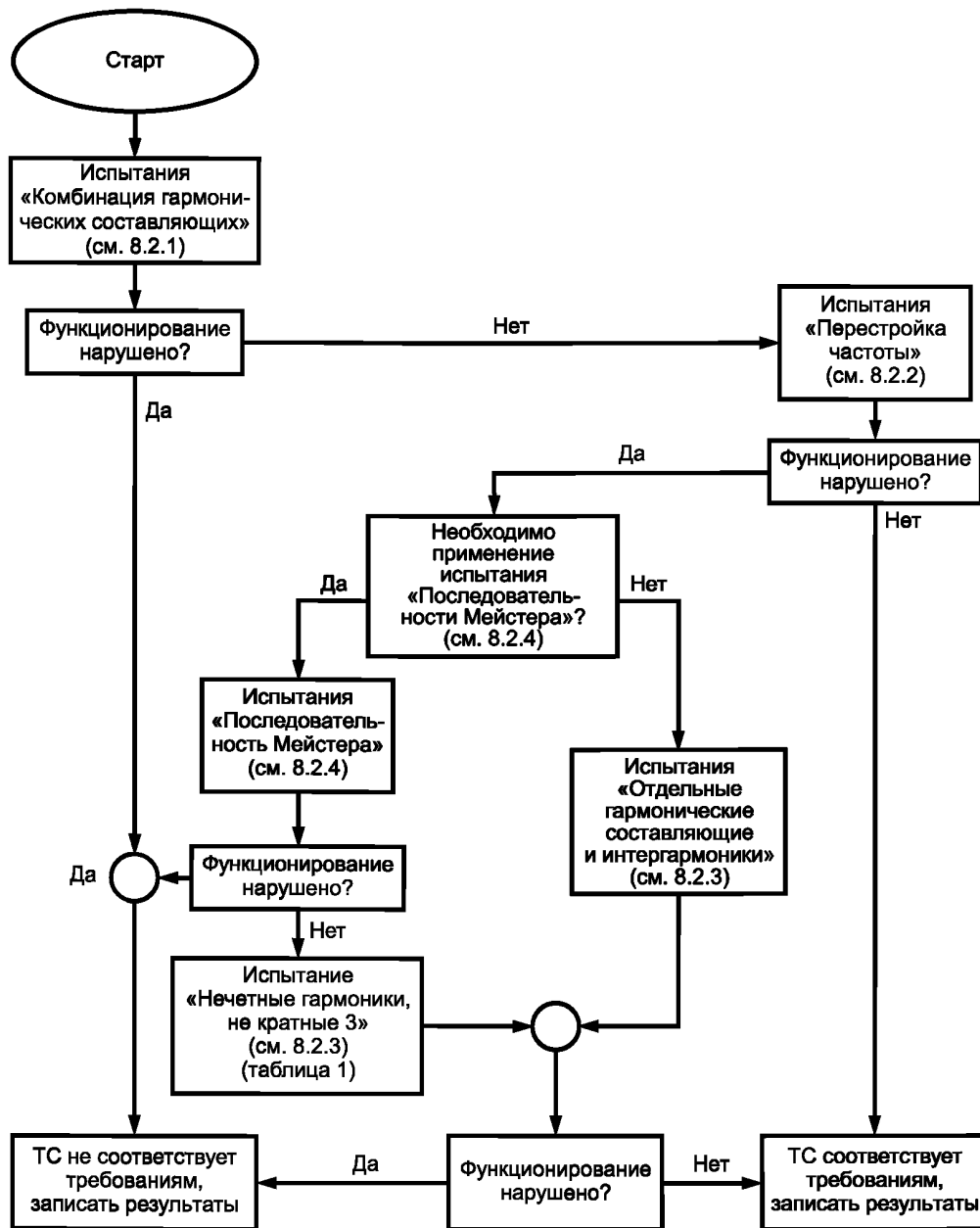
Рисунок 4 — Рекомендуемый алгоритм проведения испытаний (класс электромагнитной обстановки 3)
