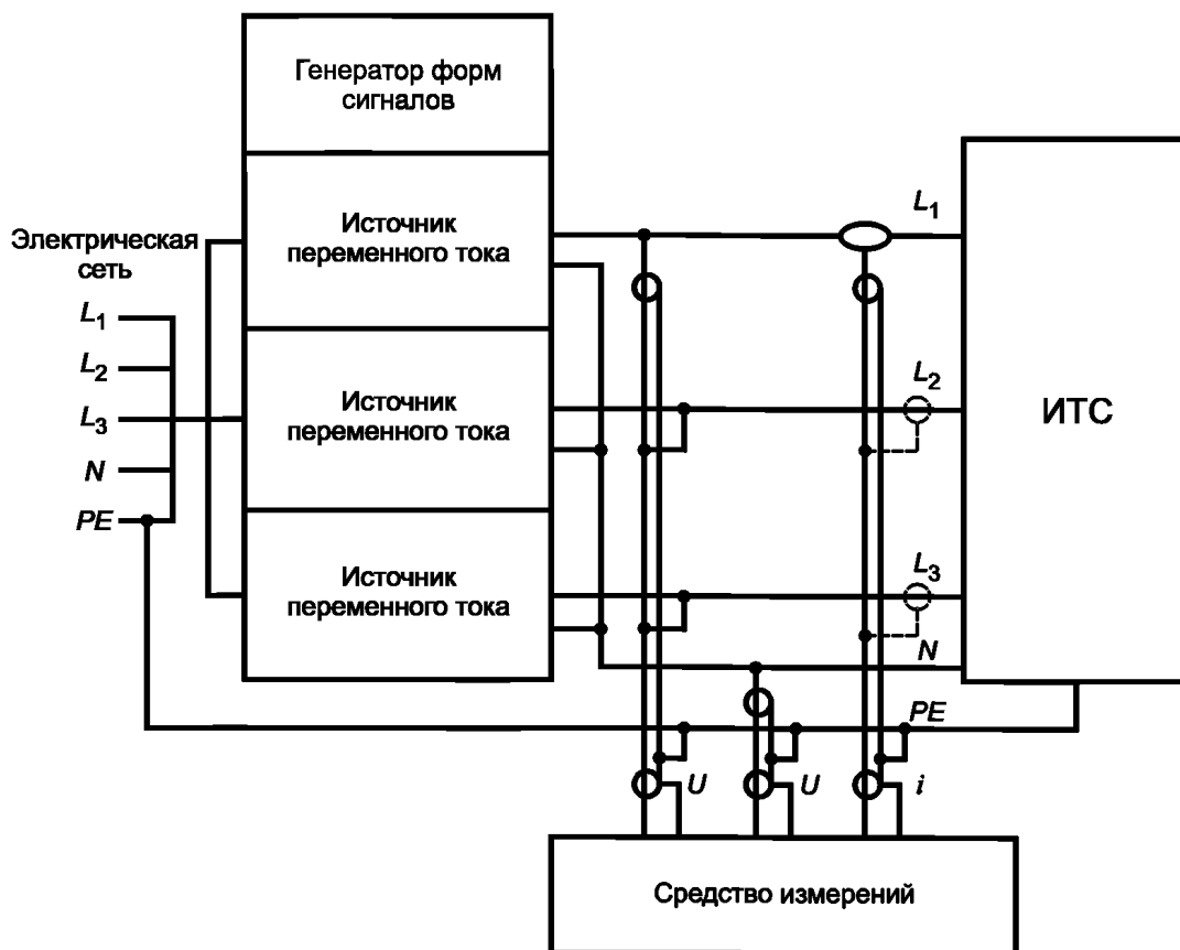
Рисунок 1 — Схема испытательной установки с использованием однофазного ИГ
