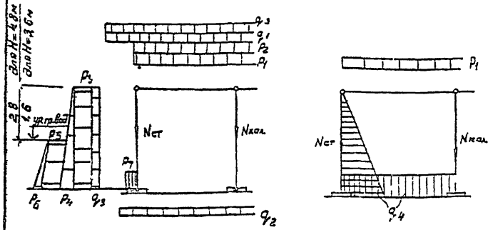
Рис. 1 Схемы расчетных сочетаний нагрузок
