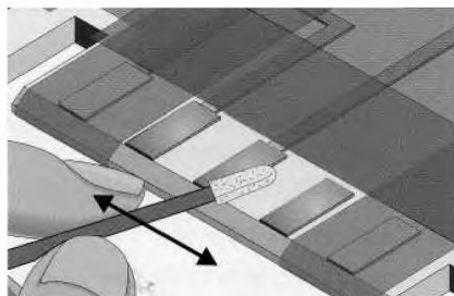
Рисунок 36 с – Удаление припоя
