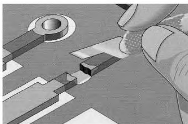
Рисунок 26 а – Удаление ножом участка печатного проводника
