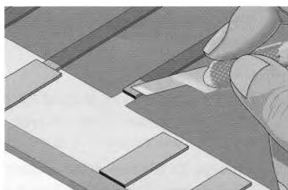
Рисунок 35 а – Удаление поврежденного концевого контакта
