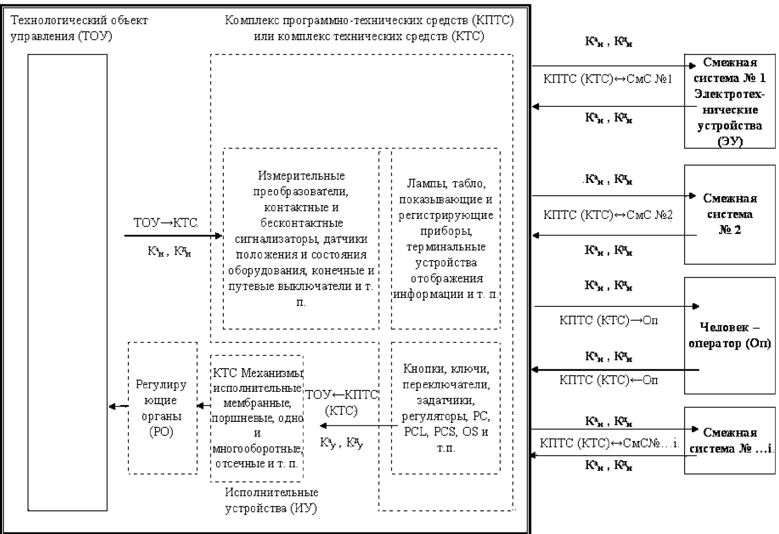
Схема автоматизированного технологического комплекса (АТК)
