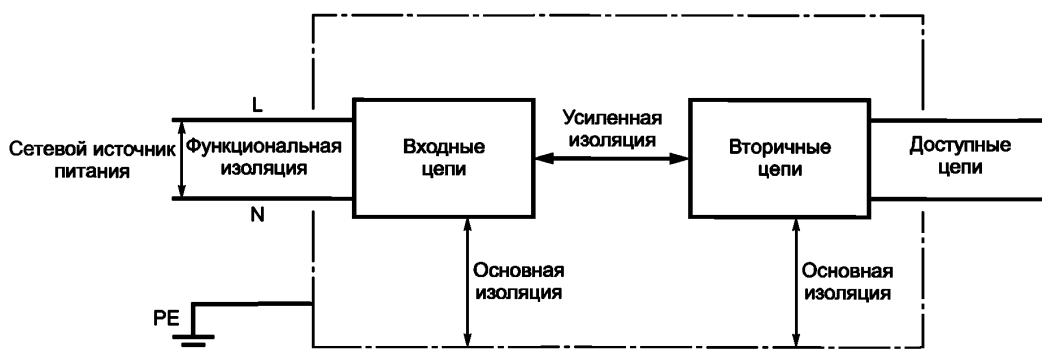
Рисунок 5а — Пример 1 — Упрощенная схема изоляционной системы, содержащей функциональную, основную и усиленную/двойную изоляцию для оборудования класса I
