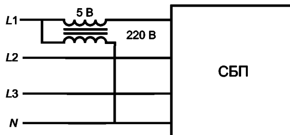
Рисунок D.1 — Амплитудная несимметрия
