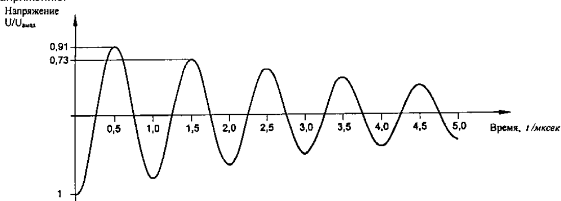
Рисунок 5 - Затухающее переменное напряжение ( f_r = 1 кГц, D_f = 0,2 )
