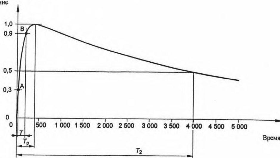
Рисунок 3 - Аперiodический коммутационный импульс
