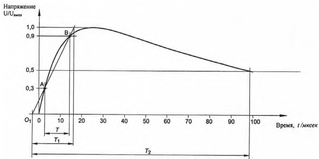
Рисунок 1 – Аперриодический грозовой импульс
