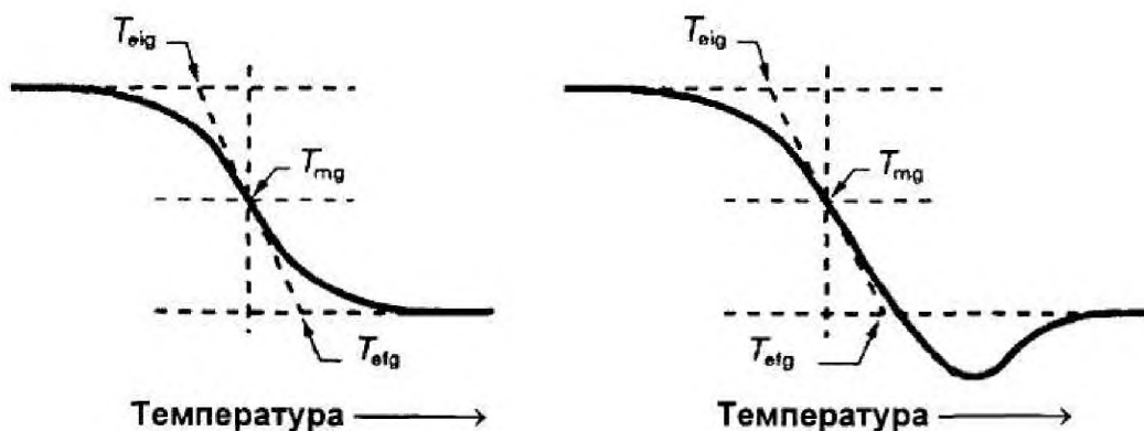
Рисунок 1 – Пример определения температуры стеклования по кривой ДСК
