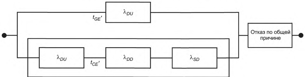
Рисунок В.11 — Структурная схема надежности для архитектуры 1oo2D
