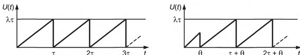
Рисунок В.19 — Мгновенная неготовность U(t) отдельного периодически проверяемого элемента
