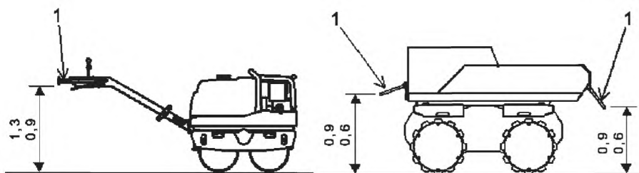
а) Каток с ручным управлением
