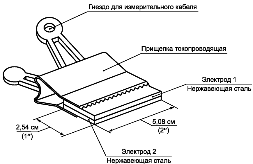
Рисунок 7 — Зажимы/электроды для испытания висящей одежды
