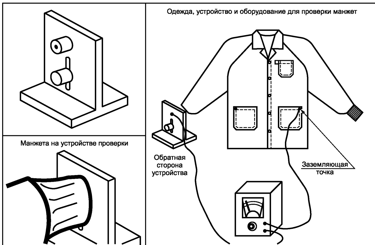
Рисунок 10 — Испытания манжет заземляемой одежды
