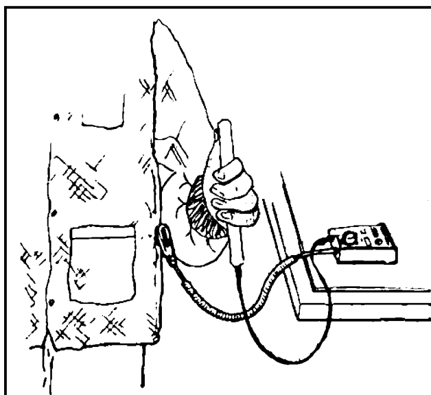
Рисунок 11 — Испытательная сборка — сопротивление системы заземляемой одежды (использование измерителя и ручного электрода при испытании надетой заземляемой одежды)
