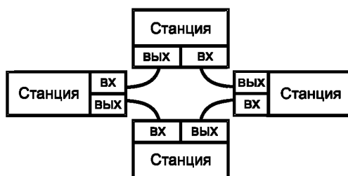
Рисунок 4 — Топология «кольцо»
