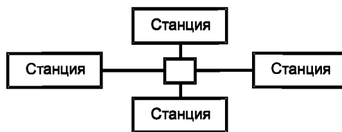
Рисунок 3 — Топология «звезда»
