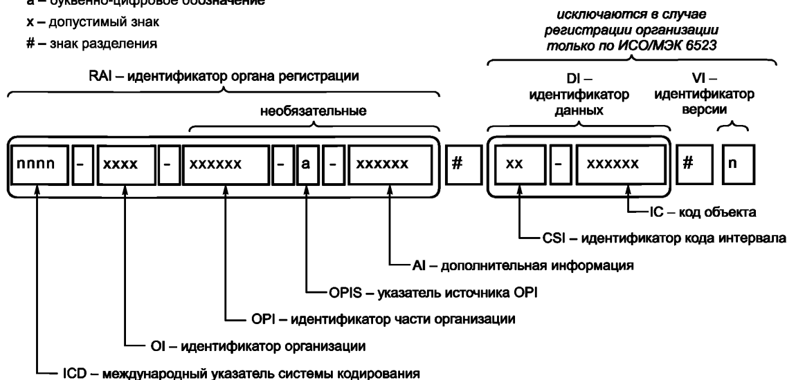
Рисунок 1 — Структура идентификатора IRDI
