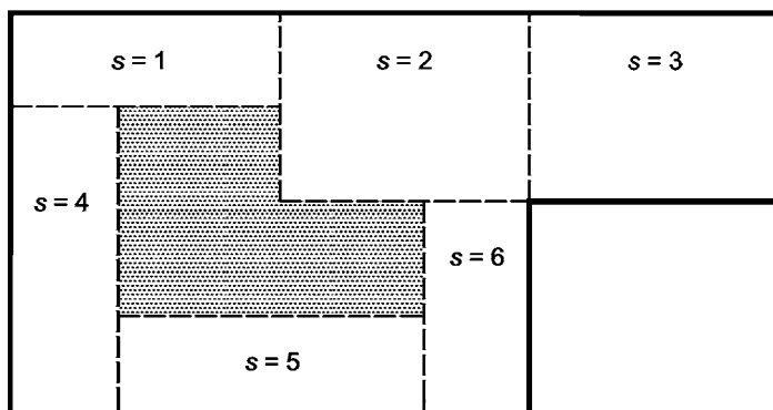
Рисунок D.2 — Пример помещения неправильной формы и его разделения на подпространства
