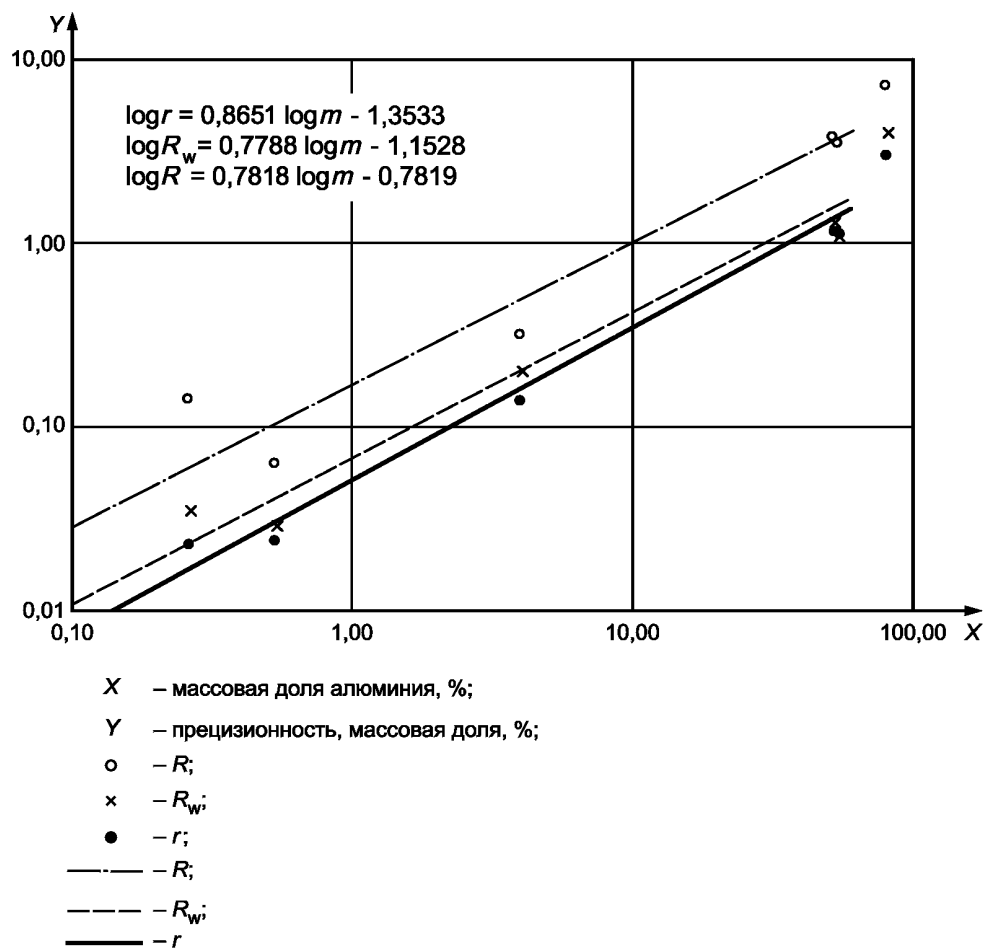
Рисунок С.3 — Данные прецизионности для определения алюминия
