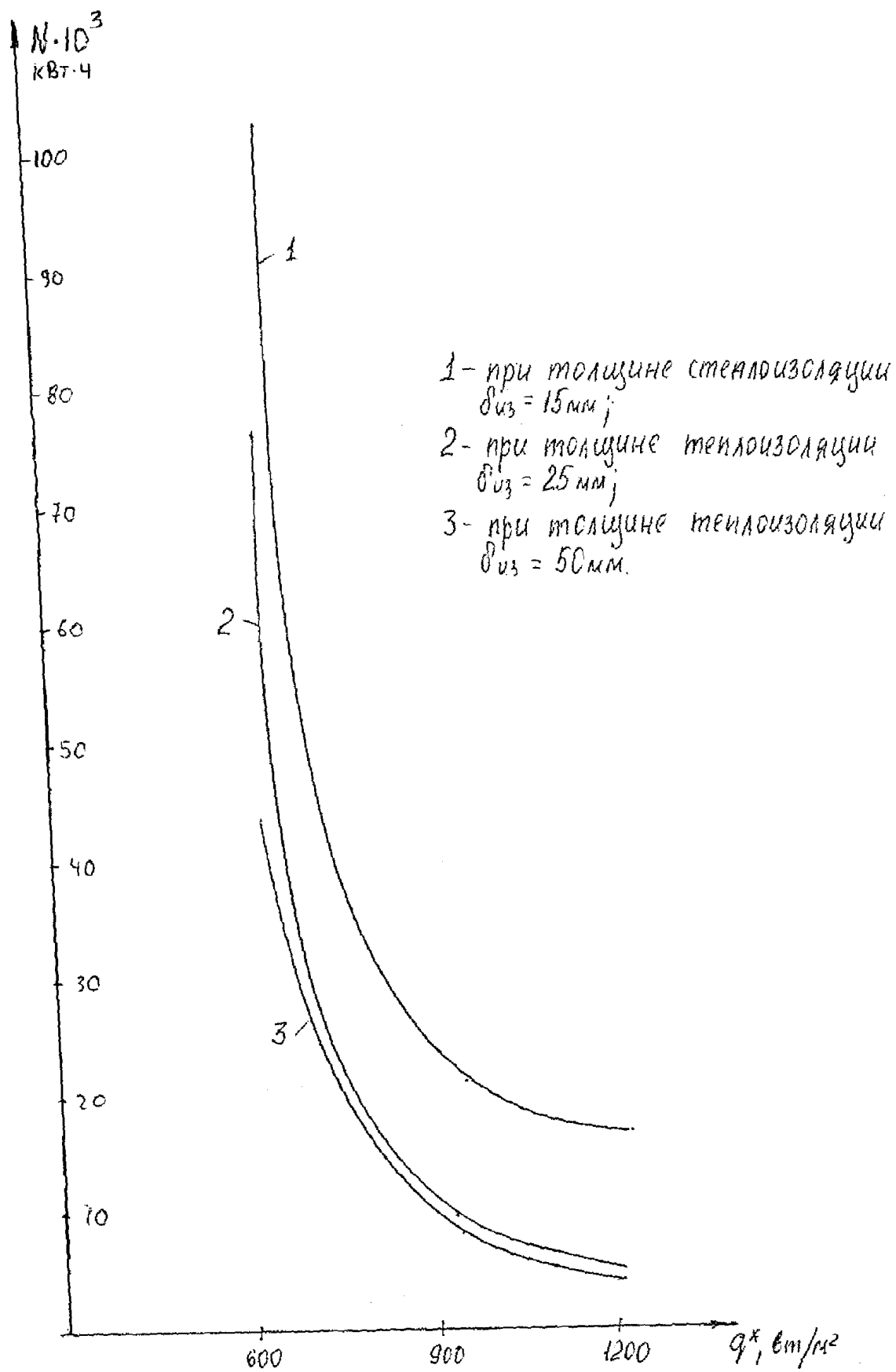
Рис. 4. Зависимость затрат электроэнергии от мощности электрообогрева.
