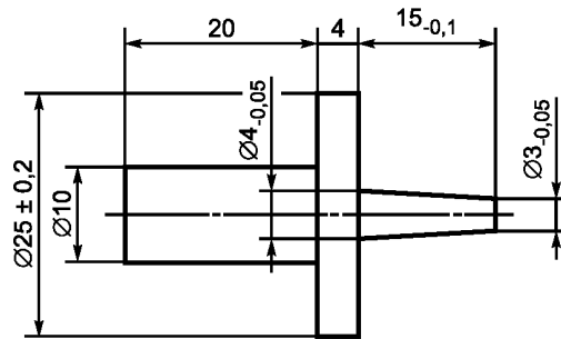
Рисунок 2 – Испытуемый стержень
