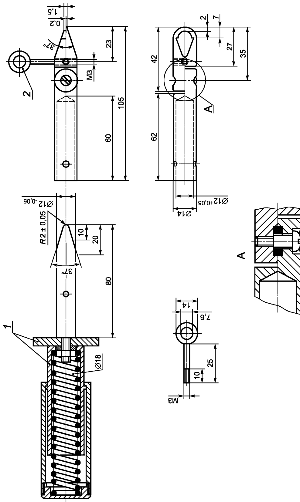
Рисунок 10 – Испытуемый ноготь
