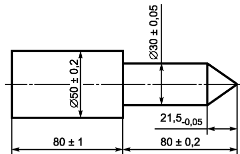
Рисунок 3 – Испытуемый щуп
