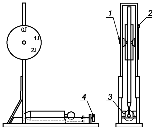
1 – подшипник; 2 – фиксирующийся указатель; 3 – спусковое основание; 4 – спусковой механизм
