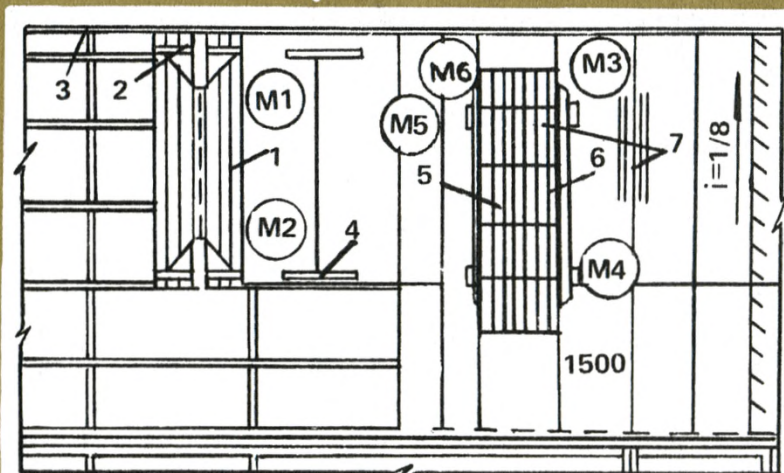
СХЕМА ОРГАНИЗАЦИИ РАБОЧЕГО МЕСТА 1 — укладываемая панель; 2 — траверса; 3 — крайние прогоны; 4 — деревянные рейки; 5 — пакет с панелями; 6 — поддон; 7 — прокладки; M1—M6 — рабочие места монтажников
