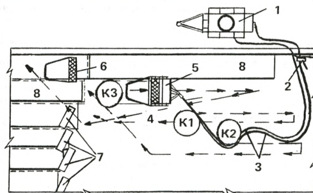
СХЕМА ОРГАНИЗАЦИИ РАБОЧЕГО МЕСТА 1 — передвижная кровельная установка ПКУ-35М; 2 — регистр для распределения лака на два звена; 3 — материальные шланги; 4 — удочка-распылитель; 5 — каток-раскатчик; 6 — каток для прикатки наклеенного рулонного ковра; 7 — рулоны рубероида, подготовленные к наклейке; 8 — наклеенный рулонный ковер; К1, К2, К3 — рабочие места кровельщиков (стрелками показано направление движения кровельщиков)
