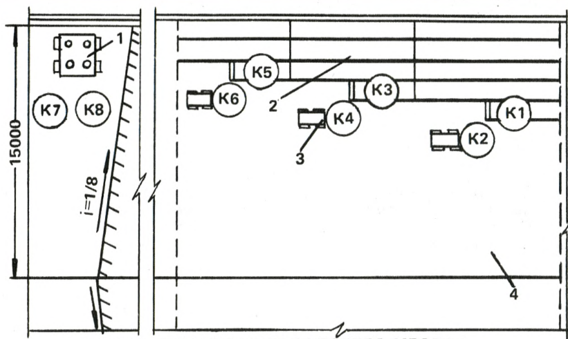
СХЕМА ОРГАНИЗАЦИИ РАБОЧЕГО МЕСТА 1 — площадка для приема материалов; 2 — наклеиваемые рулоны; 3 — тележка с битумной мастикой; 4 — огрунтованное основание; К1—К8 — рабочие места кровельщиков
