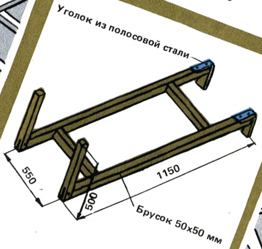
Рис. 5. Подставка
