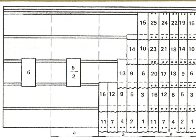
СХЕМА УКЛАДКИ ЛИСТОВ НА ОДНОЙ ЗАХВАТКЕ (цифрами обозначена последовательность укладки)
