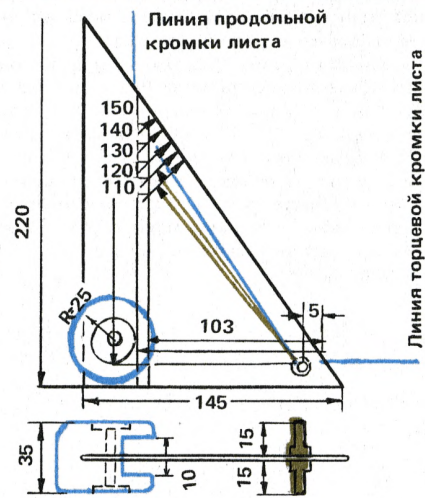
Рис. 6. Угольник
