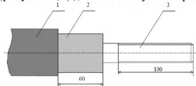
1 – наружная оболочка, 2 – изоляция, 3 – токопроводящая жила а) разделка кабеля с однопроволочной жилой при тяжении за жилу
