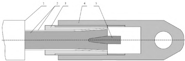
1- кабель, 2 – жила кабеля, 3 – втулка, 4 – приспособление для тяжения, 5 – клин в) клиновый захват для тяжения кабеля с однопроволочной жилой Рисунок 4 - Протяжка кабеля с помощью концевое и клинового захвата
