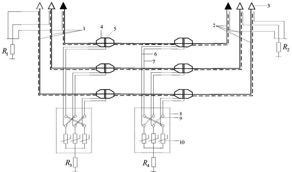
1- жилы кабелей, 2 – экраны кабелей, 3 – концевые муфты, 4 – транспозиционная муфта, 5 – изолятор транспозиционной муфты, 6 – жила транспозиционного кабеля, 7 – экран транспозиционного кабеля, 8 – коробка транспозиции, 9 – шины транспозиции, 10 – защитные аппараты (ограничители перенапряжений)
