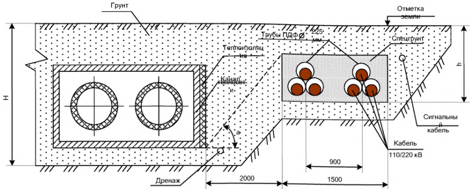
Рисунок И.4 – Пример прокладки кабелей 110 (220) кВ при прохождении трассы КЛ параллельно теплосети
