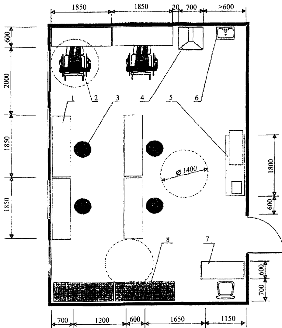
1 – верстак столярный; 2 – рабочее место инвалида; 3 – табурет с регулируемым сиденьем; 4 – стол с выгжкой; 5 – верстак с деревообрабатывающим станком и циркулярной пилой; 6 – мойка; 7 – стол мастера; 8 – стеллаж производственный
