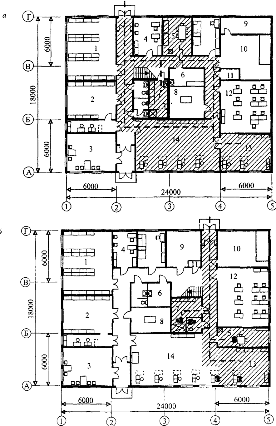
a – аналог; б – перепланировка;
