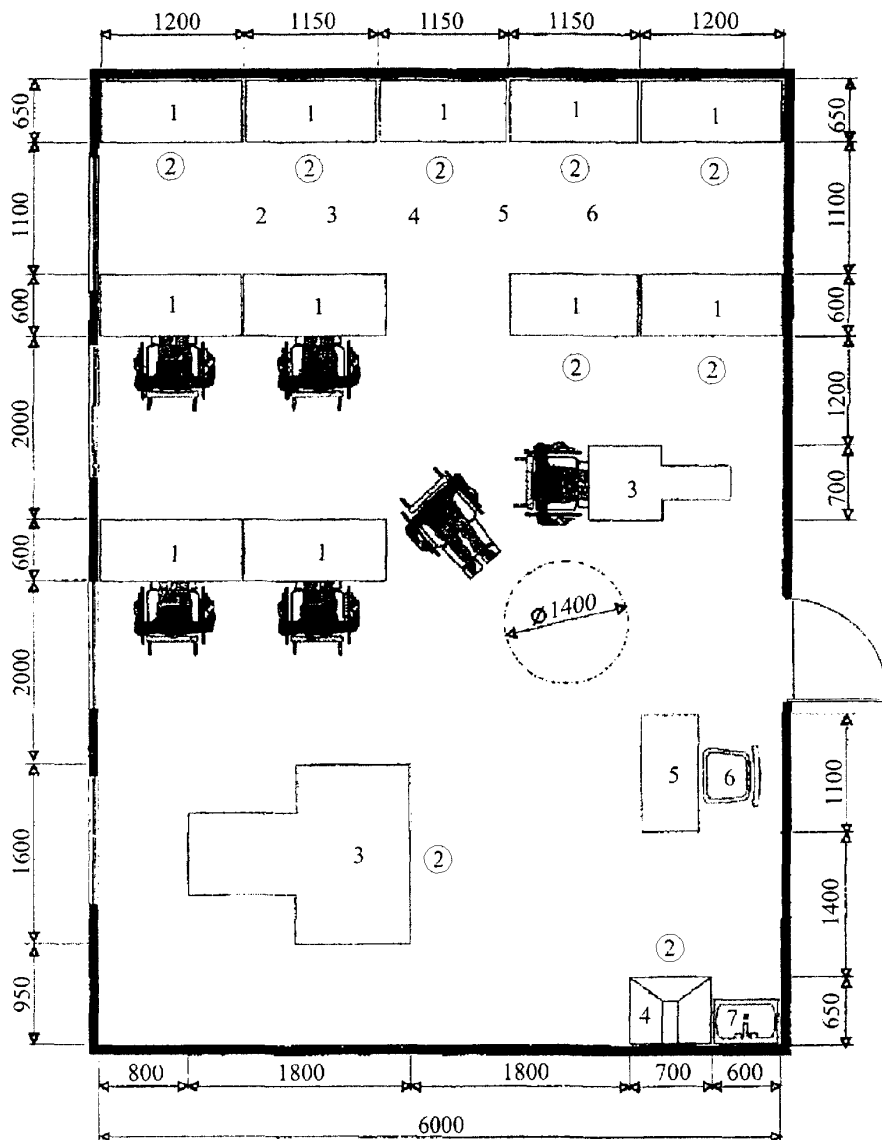
1 – стол рабочий; 2 – табурет с регулируемым сиденьем; 3 – проволочно-швейный аппарат; 4 – клееварка; 5 – стол мастера; 6 – стул 7 – мойка
