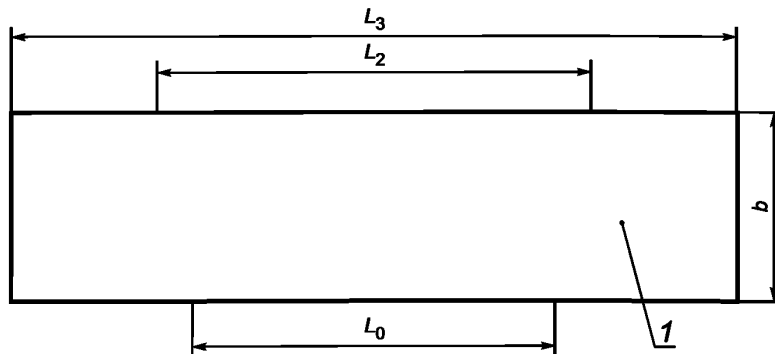
Рисунок 1 — Образец-полоска (метод А)
