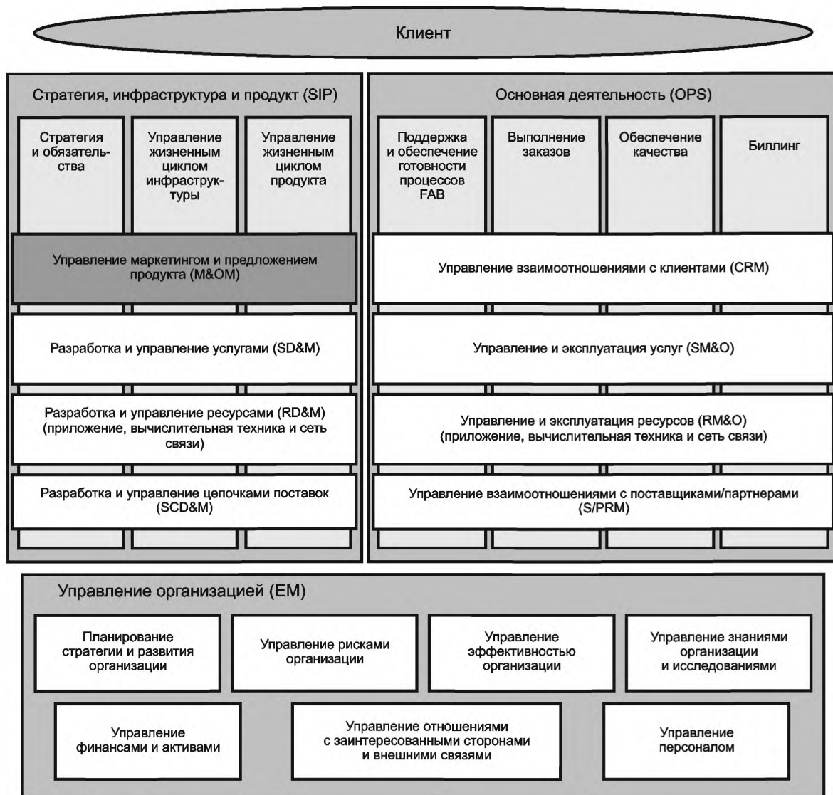
Рисунок 1 — Структура уровня 1 общей структуры бизнес-процессов eTOM
