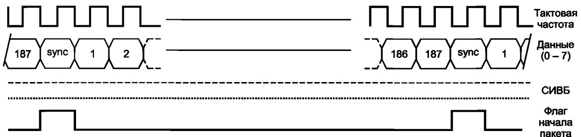
Рисунок 4 — Формат передачи пакетов 188 байт
