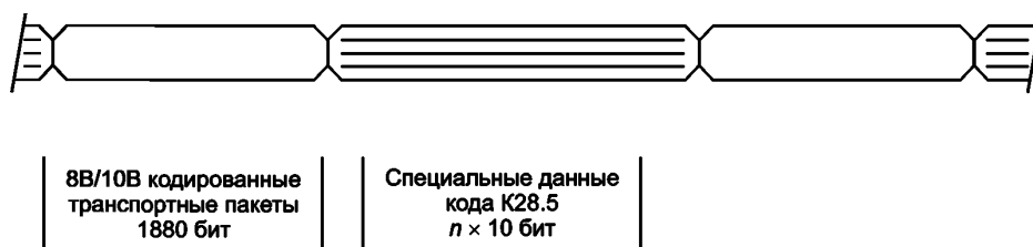
Рисунок 21 — Формат передачи пакетных данных
