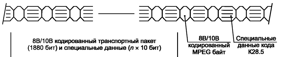
Рисунок 22 — Формат передачи отдельных байт
