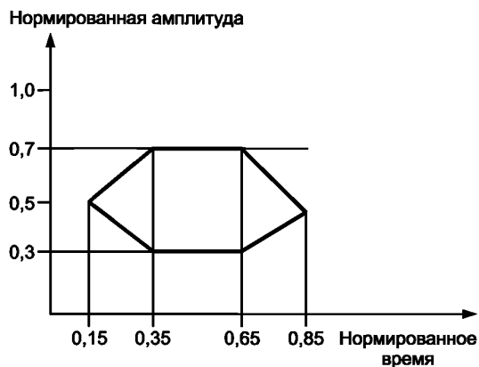
Рисунок 20 — Маска глазовой диаграммы передатчика при измерении джиттера
