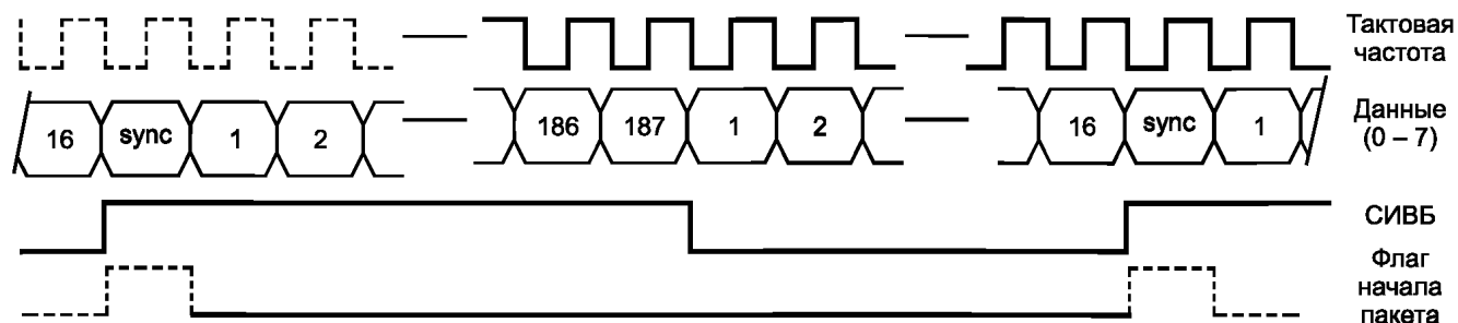
Рисунок 5 — Формат передачи пакетов 204 байта
