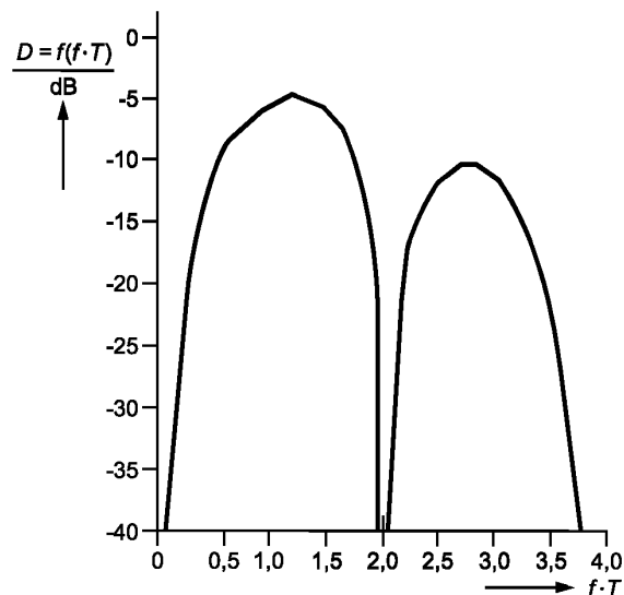
Рисунок 13 — Спектральные плотности инверсного биполярного кода БВН
