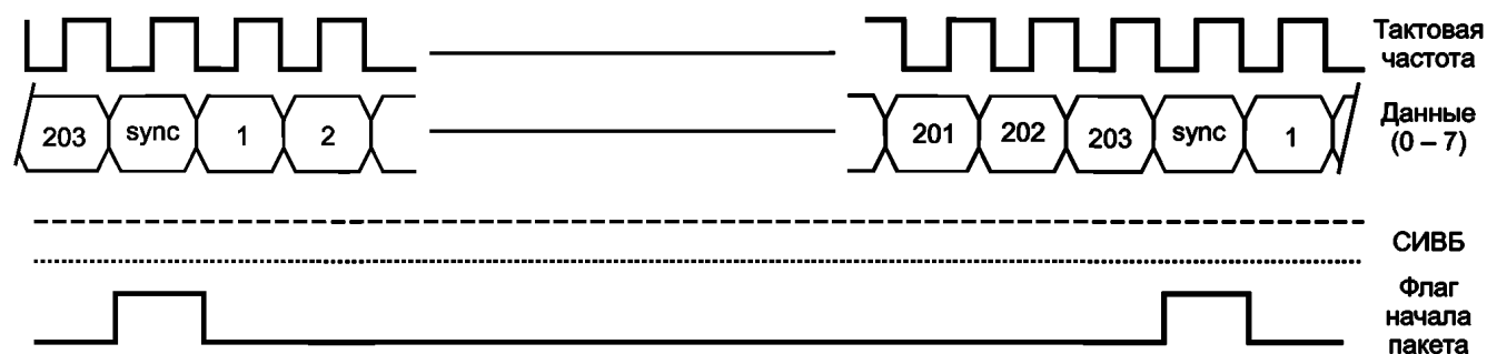
Рисунок 6 — Формат передачи пакетов с кодированием Рида-Соломона (204 байта)
