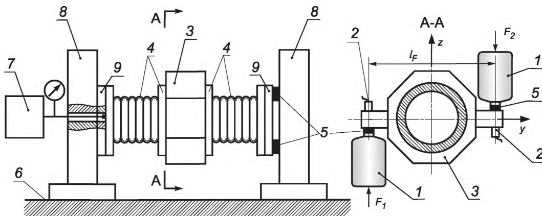
1 — вибровозбудитель; 2 — датчик вибрации; 3 — промежуточная конструкция; 4 — испытываемые упругие вставки с жидкостью; 5 — датчик силы; 6 — жесткий фундамент; 7 — система подачи жидкости; 8 — опора; 9 — заглушка
