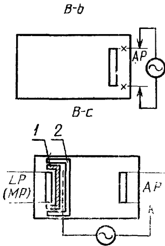
1 — ОСНОВНАЯ ИЗОЛЯЦИЯ, 2 — ДОПОЛНИТЕЛЬНАЯ ИЗОЛЯЦИЯ
