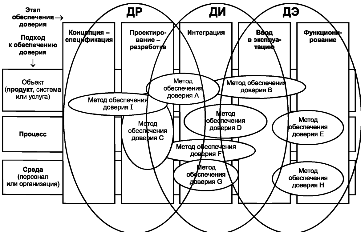
Рисунок 5 — Обеспечение доверия
