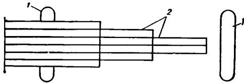
Рис. 5. Схема надвигки многостенчатых стальных пролетных строений
