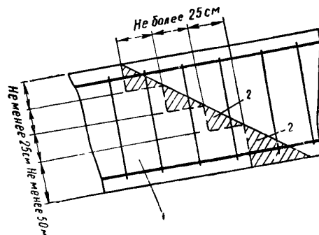
Рис. 8. Обработка рабочего шва элемента при значительной высоте его
