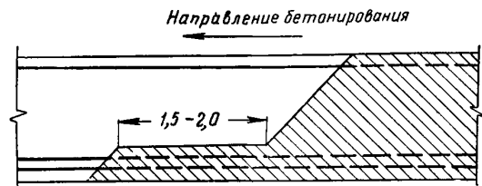
Рис. 7. Схема бетонирования балочных конструкций
