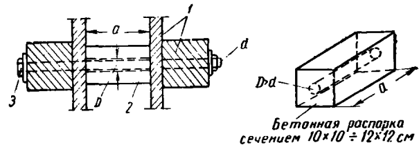
Рис. 6б. Бетонная распорка
