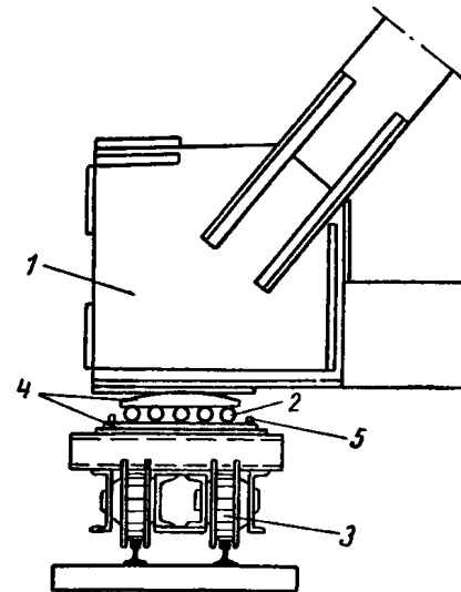
Рис. 2. Поперечная перекатка на специальных тележках
