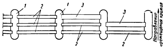
Рис. 4. Последовательность монтажа сборных сводов 1 — опоры; 2 — смонтированные своды; 3 — кружала
