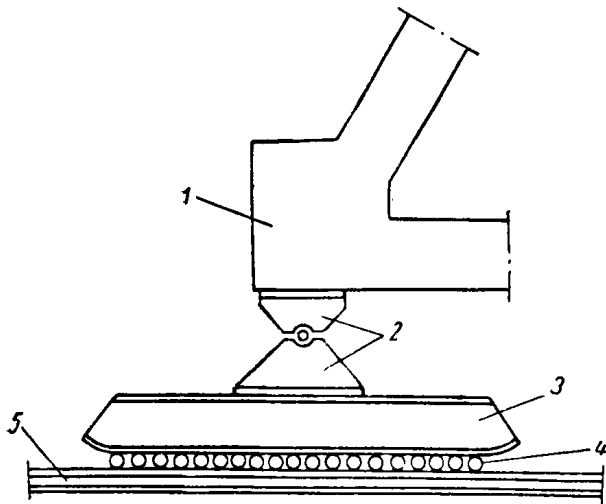
Рис. 1. Опираие опорного узла пролетного строения на накаточные пути при продольной надвигке на плаву
