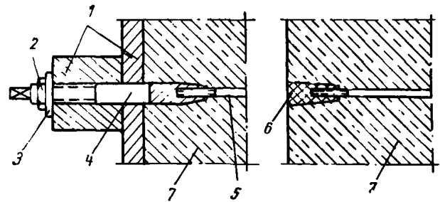
Рис. 6а. Стяжка со съемным наконечником
