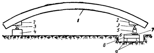
Рис. 3 Схема опирания концов пролетного строения (блока) при подъеме его с поворотом вокруг одного из концов конструкции
