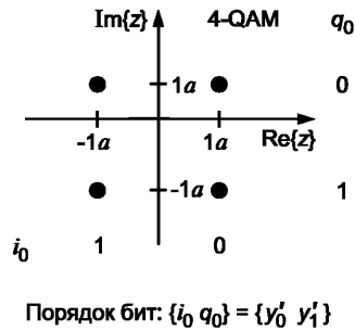
Рисунок 6 — SM 4-QAM отображение с соответствующей битовой комбинацией
