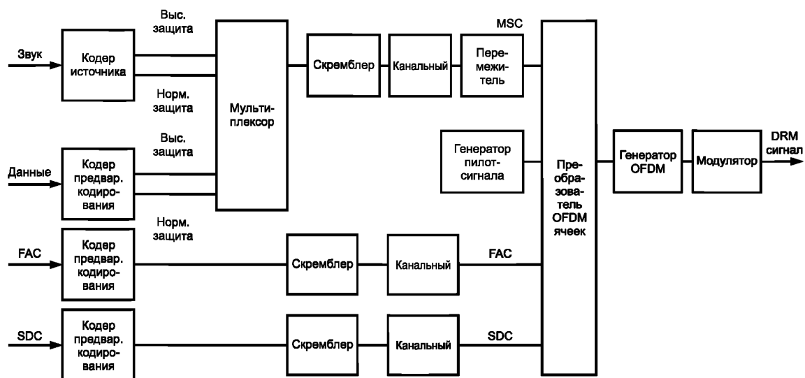
Рисунок 1 — Структурная схема передающей части системы DRM
