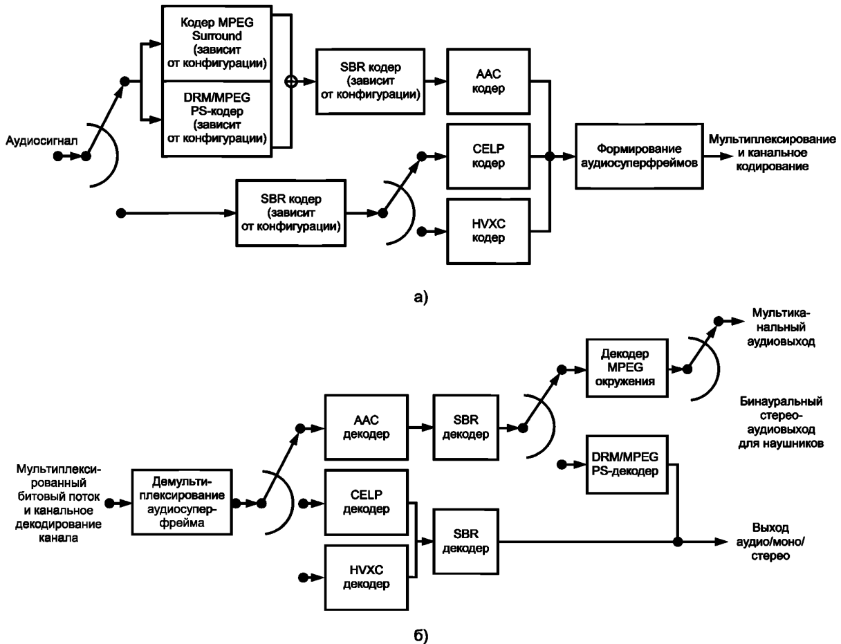
Рисунок 2 — Кодирование (а) и декодирование (б) источников аудиосигналов
