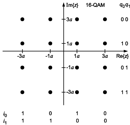
Рисунок 5 — SM 16-QAM отображение с соответствующей битовой комбинацией
