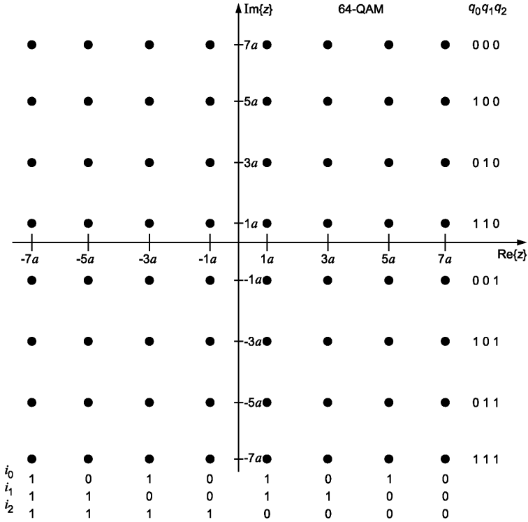
Рисунок 4 — SM 64-QAM отображение с соответствующей битовой комбинацией
