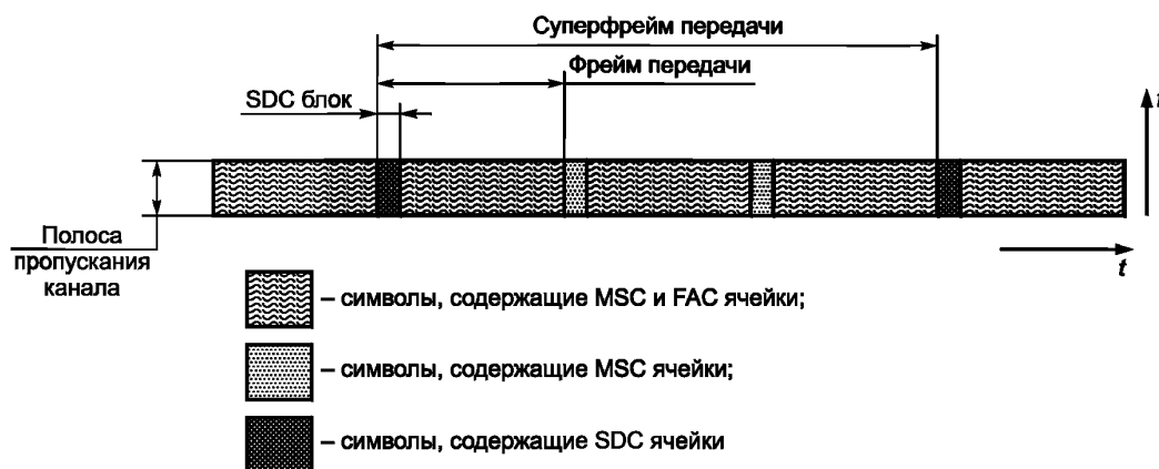
Рисунок 9 — Частотно-временное расположение FAC и SDC сигналов
