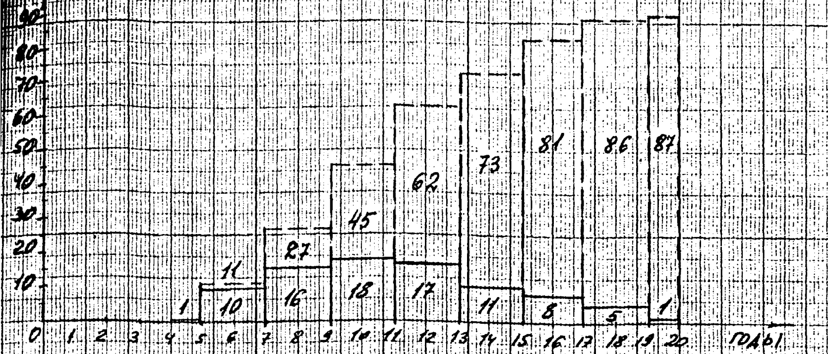
Рис. 2.1. Гистограмма количества отказов в зависимости от наработки (для участка L=400 км Г/П БУХАРА-УРАЛ).
