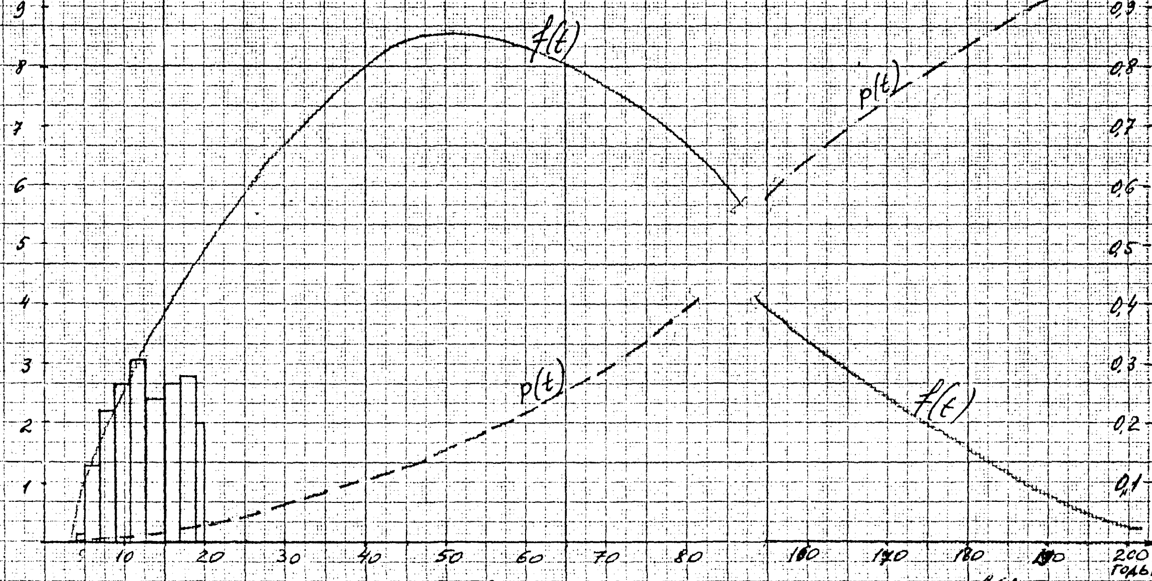
Рис. Зная плотность вероятности времени до коррозионного отказа f(t) и вероятность безотказной работы p(t) , построены с учетом замеченных углублений.
