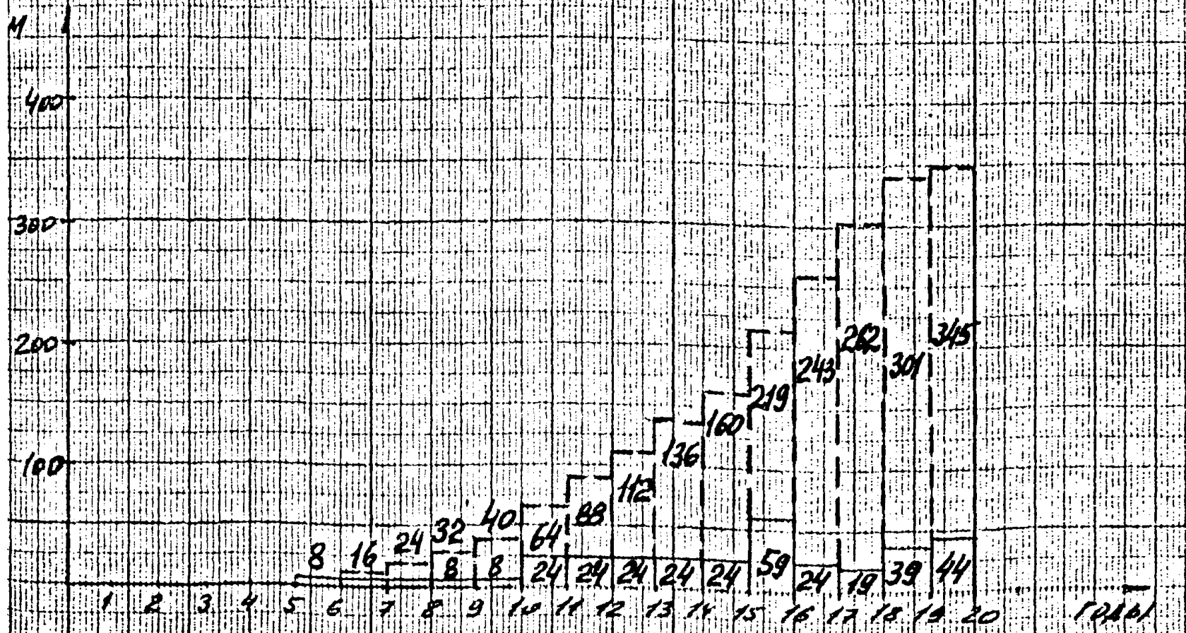
Рис. 2.2. Гистограмма замены участков трубопровода в результате капремонта.
