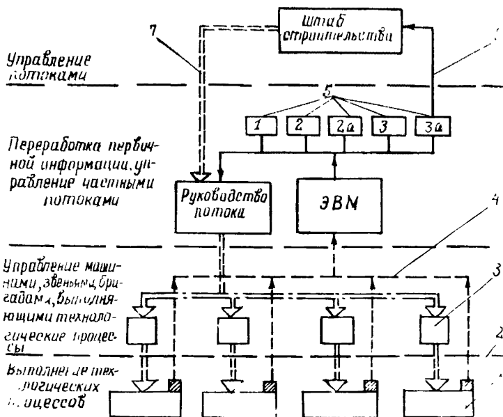
Рис.2. Схема информационных потоков и управляющих воздействий АСУ ТП трубопроводостроительного комплекса:
