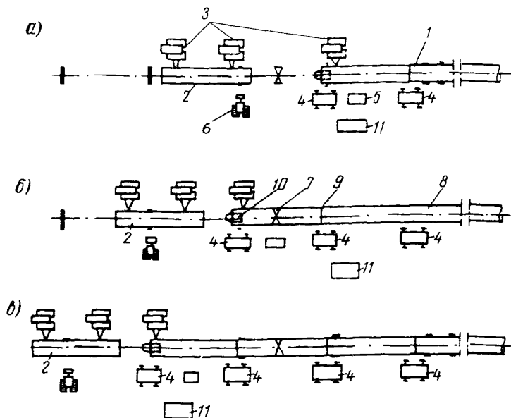
Рис.4. Монтаж прямолинейного участка надземного трубопровода: а - в-последовательность монтажа; I-смонтированный трубопровод; 2-собираемая секция; 3-трубоукладчики Т3560 или К-594; 4-сварочные агрегаты СДУ-2Б; 5-сани с кислородными и пропановыми баллонами; 6-бульдозер Д-271А; 7-неподвижная опора; 8-продольно-подвижная опора; 9-грунтовая или снежная призма; 10-центратор ЦВ-142 или ЦВ-141; II-передвижной домик
