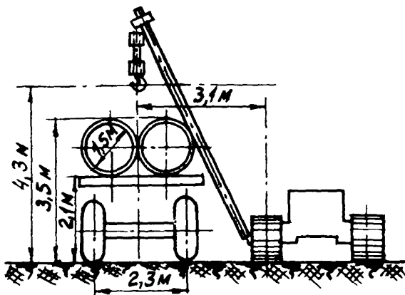
Рис.1. Схема разгрузки пакета из двух труб плетового МАЗ-543 трубоукладчиком К-594
