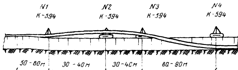
Рис.8. Размещение механизмов в колонне при укладке изолированного трубопровода
