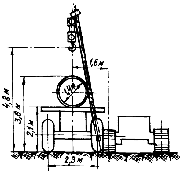
Рис.2. Схема погрузки (разгрузки) треструбой секции (36 м) на плетевоз МАЗ-543 трубоукладчиком К-594
