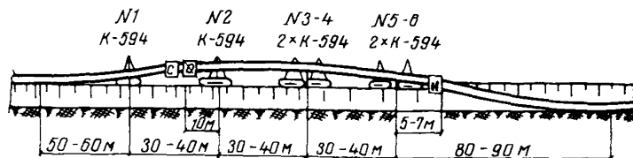
Рис.6. Размещение механизмов в колонне при укладке трубопровода \varnothing 1420 мм в условиях устойчивых грунтов
