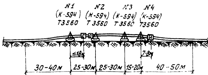
Рис. 9. Размещение механизмов в механизированной колонне при наземной прокладке трубопровода диаметром 1-20 мм;
