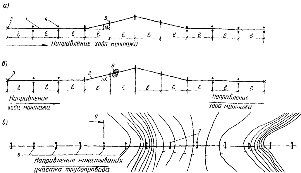
Рис.3. Схемы производства монтажных работ при надземной прокладке:
