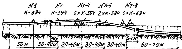
Рис.7. Размещение механизмов в колонне при укладке трубопровода \varnothing 1420 мм в условиях неустойчивых грунтов
