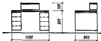
106. Стол оператора по управлению информационной аппаратурой Шифр 1-01-04-17
