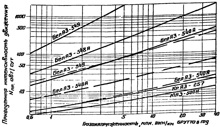
Рис 30 Номотрица для определения приведенной интенсивности движения к расчетному автомобилю БелАЗ-548. Обозначенная также, что и на Рис. 28
