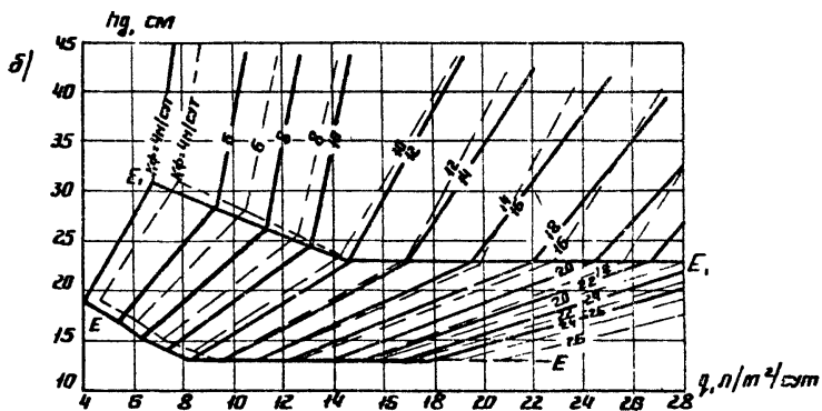
Рис. 21 График для определения толщины ограничивающего слоя при поперечном профиле дорожной суежды с индексом D и путн. фильтрации Юм
