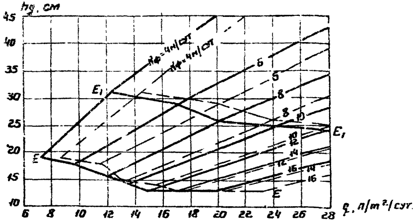
Рис. 7 График для определения толщины дренажного слоя при поперечном профиле дорожной одежды с индексом В и Г и пути фильтрации 4 м
