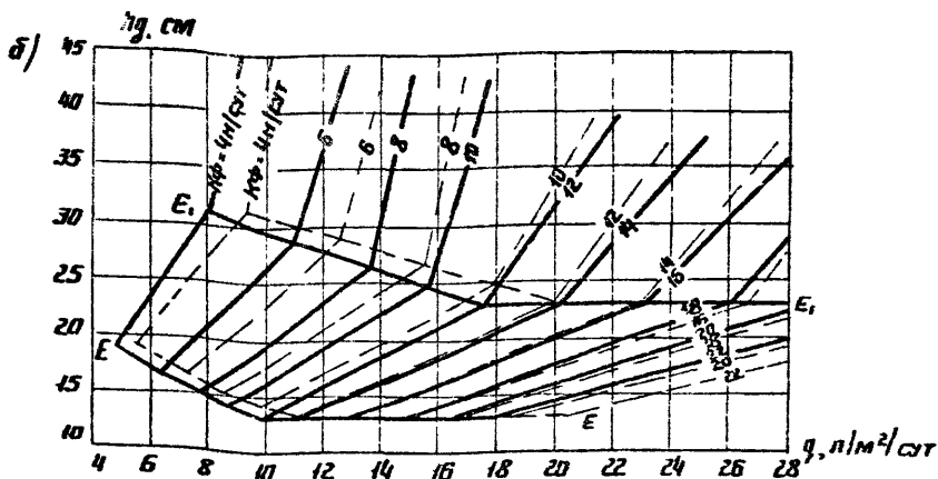
Рис. 20 График для определения толщины дренирующего слоя при поперечном профиле дорожной одежды с индексом D и пути фильтрации 9 м.
