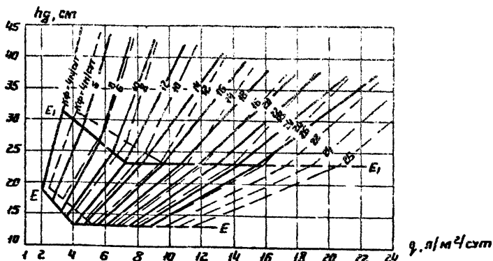
Рис. 13 График для определения толщины дренажного слоя при поперечном профиле дорожной одежды с индексом \Gamma и пути фильтрации 10n Обозначения те же, что и на рис. 7
