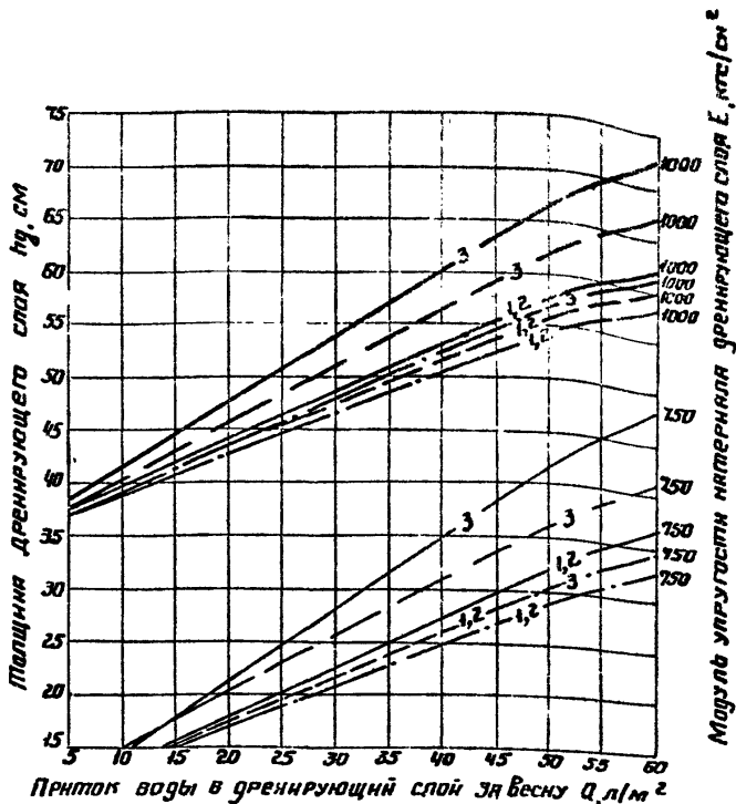
Рис. 3 График для определения толщины дренирующего слоя основания h_d , из мелкого песка при поперечном профиле проезжей части с индексом Б.
