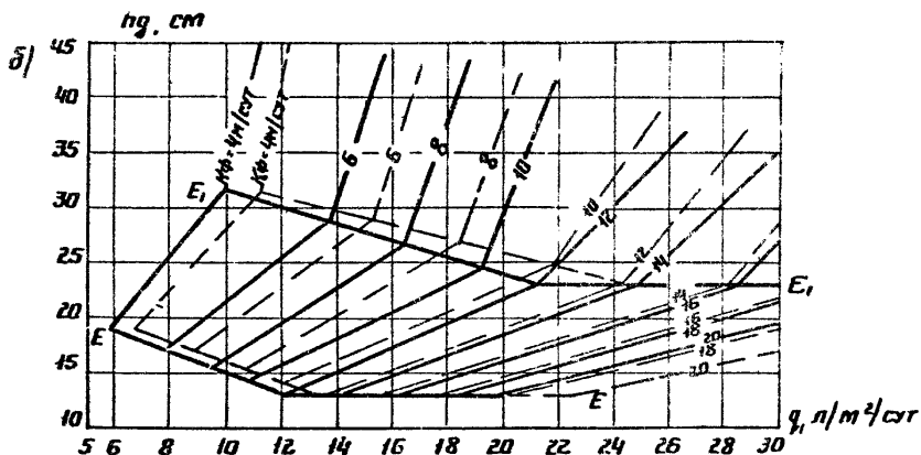
Рис. 19 График для определения толщины дренарующего слоя при поперечном профиле дорожной одежды с индексом D и пути фильтрации 8 м.
