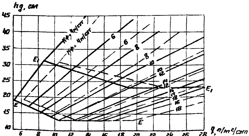
Рис. 8 График для определения толщины дренажного слоя при поперечном профиле дорожной одежды с индексом В и Г и пути фильтрации 5 м
