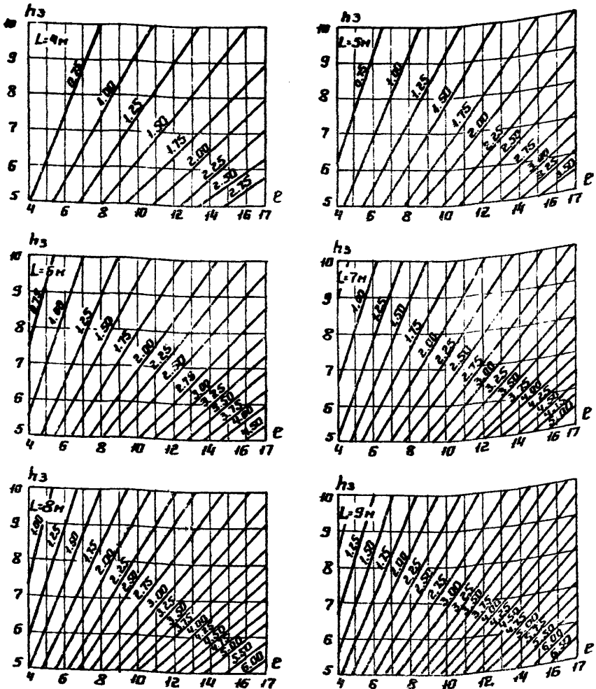
Рис. 27 Графики для определения расстояния между трапециевидными воронками (поперечный профиль дорожной одежды с индексом В)
