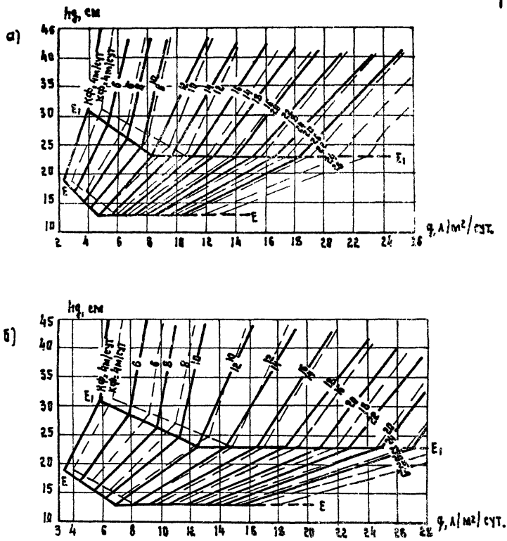
Рис. 22 График для определения толщины дренажного слоя при поперечном профиле дорожной одежды с индексом A и пути фильтрации L м.
