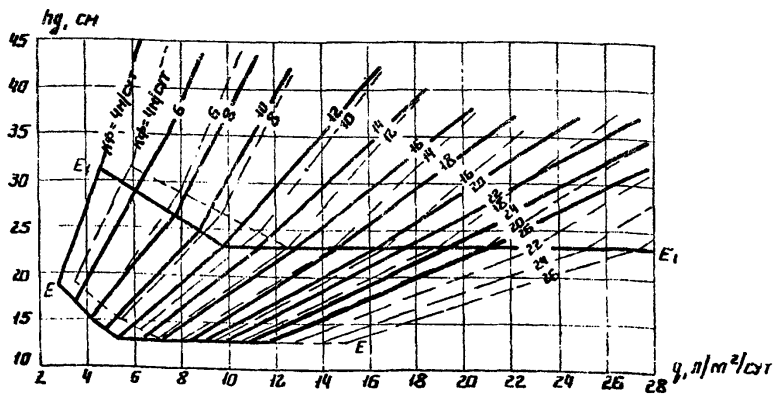
Рис. 11 График для определения толщины дренажного слоя при поперечном профиле дорожной одежды с индексом n в \Gamma и пути фильтрации 8 м. Обозначения те же, что и на рис. 7.
