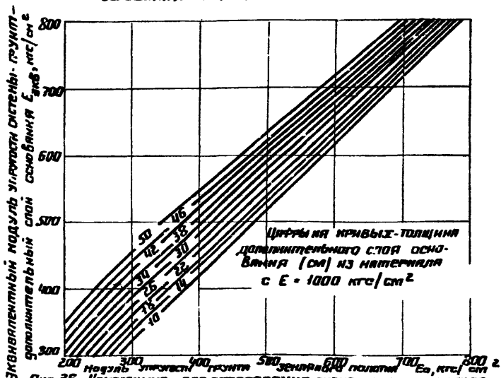
Рис. 36. Номаграмма для определения эквивалентного модуля упругости системы грунт-дополнительный слой основания при расчетном автомобиле БелАЗ-548
