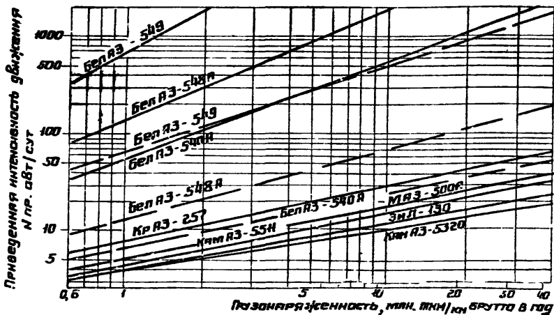
Рис. 29 Номотрия для определения интенсивности движения к расчетному автомобилю БелАЗ - 540
