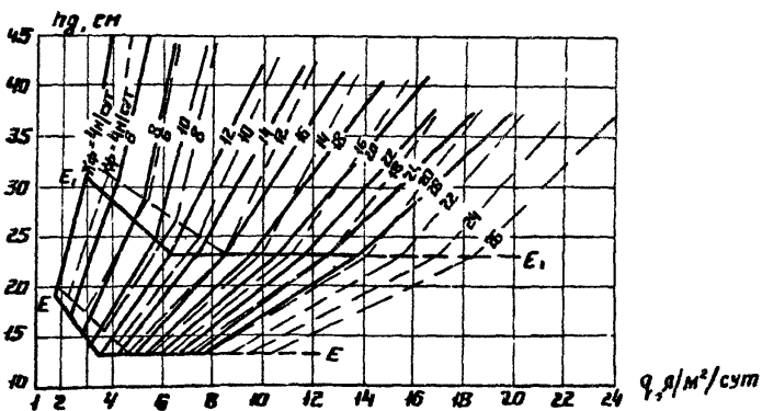
Рис. 14 График для определения толщины дренажного слоя при поперечном профиле дорожной одежды с индексом \Gamma и пути фильтрации 5n Обозначения те же, что и на рис. 7
