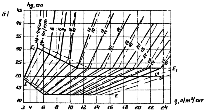
Рис 23 График для определения толщины дренажующего слоя при поперечном профиле дорожной одежды с индексом D_n пути фильтрации 12 м
