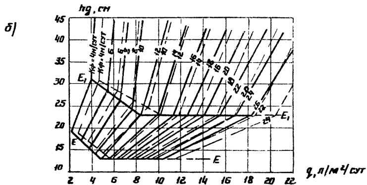
Рис. 25 График для определения толщины дренарующего слоя при поперечном профиле дорожной одежды с индексом D_n пути фильтрации 14 м а - Глубина ровика 25 см; б - Глубина ровика 45 см. Обозначения те же, что и на рис. 7
