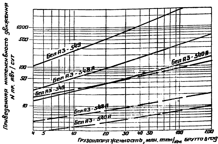
Рис 31 Номотрица для определения приведенной интенсивности движения к расчетному автомобилю БелАЗ-548 Обозначенная также, что и на Рис. 28
