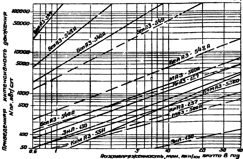
Рис. 28 Номотрия для определения приведенной интенсивности движения к расчетному автомобилю группы А
