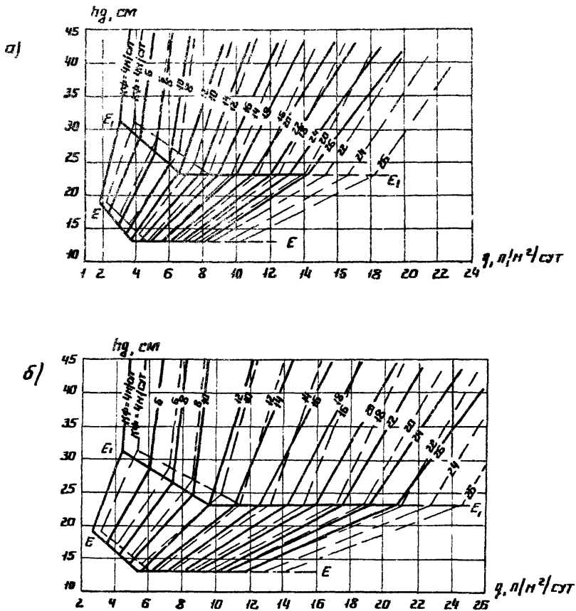
Рис 24 График для определения толщины дренажного слоя при поперечном профиле дорожной одежды с индексом \Delta и путем фильтрации 13 м а - глубина ровника 25 см; б - глубина ровника 45 см. Обозначения те же, что и на рис. 7
