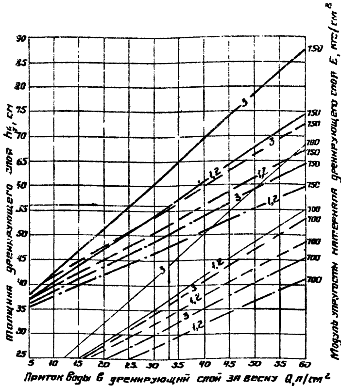
Рис. 2 График для определения толщины дренарующего слоя дорожника h_d из очень мелкого песка при поперечном профиле проезжей части с индексом Б
