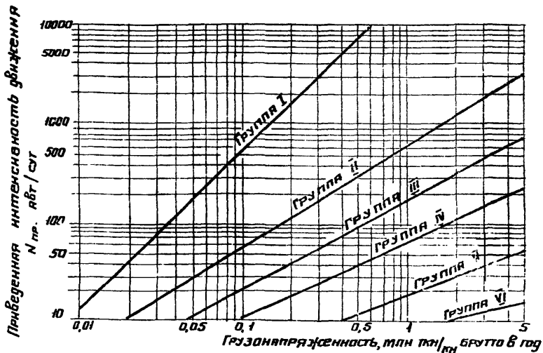
Рис. 32. Коэффициент для определения приведенной интенсивности движения погрузчиков и тележек к расчетному автомобилю группы А.
