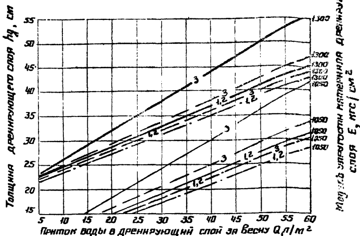
Рис. 4 График для определения толщины дренажного слоя основания h_d из песка средней крупности при поперечном профиле проезжей части с индексом B
