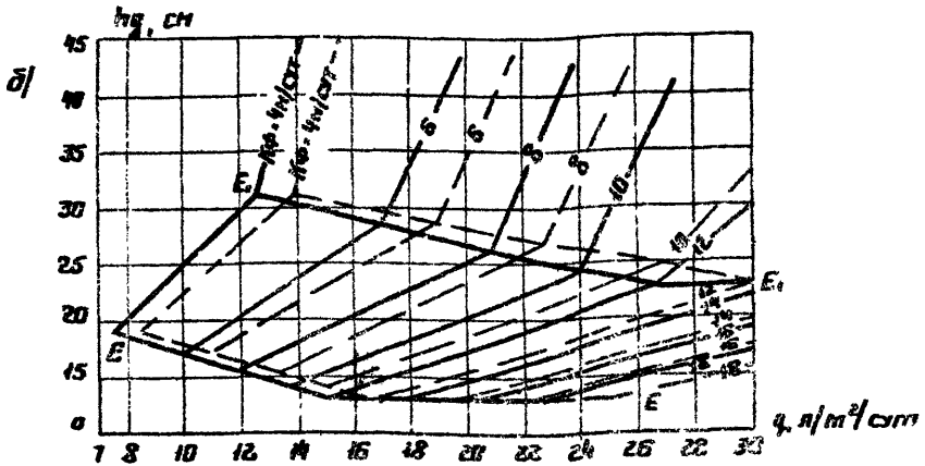
Рис. 18 График для определения толщины дренажного слоя при поперечном профиле дренажной подушки с индексом Д и пути фильтрации 7 м а - толщина ровника 25 см; б - толщина ровника - 45 см Обозначение те же, что и на рис. 7
