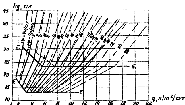
Рис. 15 График для определения толщины дренирующего слоя при поперечном профиле дорожной одежды с индексом \Gamma и пути фильтрации 12 м Обозначения те же, что и на рис. 7
