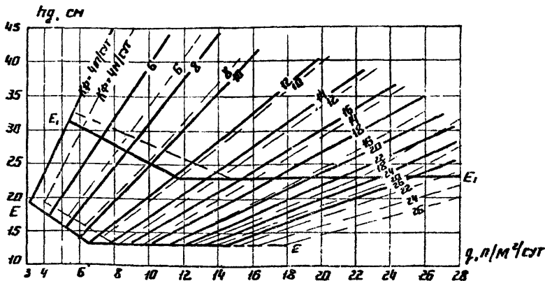
Рис. 10. График для определения толщины дренажного слоя при поперечном профиле дорожной одежды с индексами B и \Gamma и пути фильтрации 7 м. Обозначения те же, что и на рис. 7
