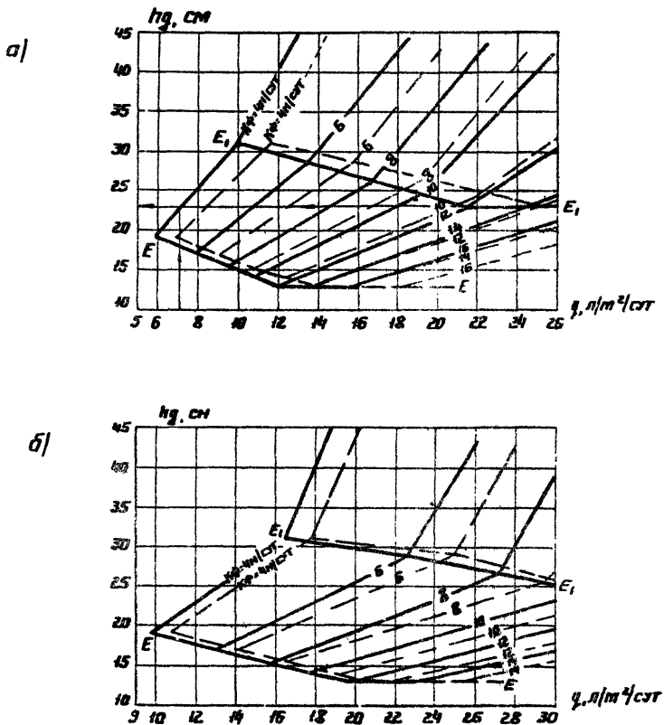
Рис.17 Пряфики для определения толщины ограничивающего слоя при поперечном профиле дорожной одежды с индексом D и пути фильтрации B а) толщина ровника 25 см; б) толщина ровника 45 см. Обозначения те же, что и на рис. 7
