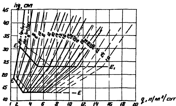
Рис. 16 График для определения толщины дренирующего слоя при поперечном профиле дорожной одежды с индексом \Gamma и пути фильтрации 13 м. Обозначения те же, что и на рис. 7
