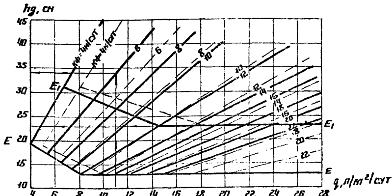
Рис. 9. График для определения толщины дренажного слоя при поперечном профиле дорожной одежды с индексами B и \Gamma и пути фильтрации B м. Обозначения те же, что и на рис. 7
