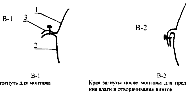
Рисунок 7 - Узел закрепления стяжек при установке скорлуп
