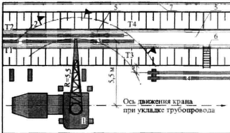
1 - кран; 2 - центратор; 3 - траверса; 4 - звено труб; 5 - непроходной канал; 6 - лестница для спуска в траншею; 7 - временное ограждение; T1 и T2, T3 и T4 рабочие места исполнителей ▲ — - граница опасной зоны
