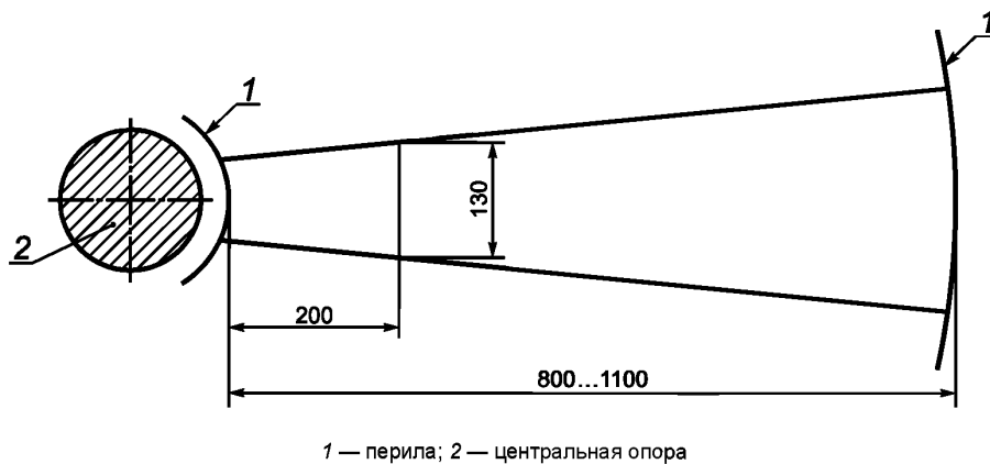
Рисунок 5 — Размеры винтовых или спиральных лестниц
