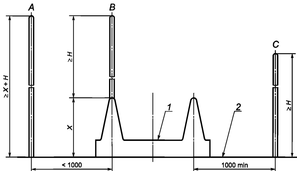
A, B, C — варианты защитных ограждений платформы: A — ограждение высотой до 1000 мм от наивысшей точки опорной поверхности на платформе; B — ограждение, расположенное по одну сторону стартового элемента; C — ограждение, расположенное на расстоянии более 1000 мм от наивысшей точки опорной поверхности на платформе; H — высота защитного ограждения; X — высота наивысшей точки опорной поверхности на платформе; 1 — стартовый элемент; 2 — платформа
