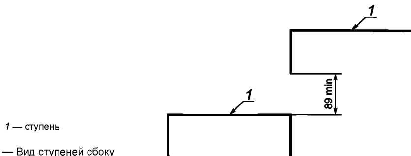
Рисунок 6 — Вид ступеней сбоку
