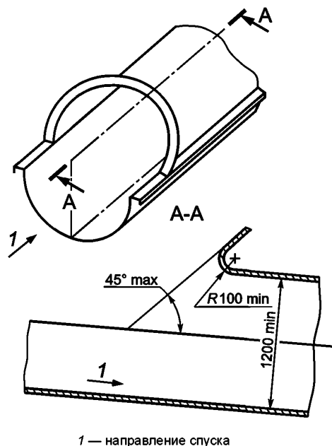
Рисунок 9 — Перекрытие начальной секции трассы спуска
